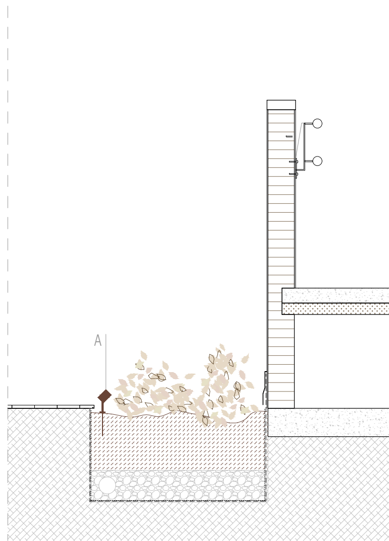
A.Focus d'exterior d'alumini negre, 35 Watts de potència amb unes dimensions de 22,5cm d'altura i 9,7cm de diàmetre
