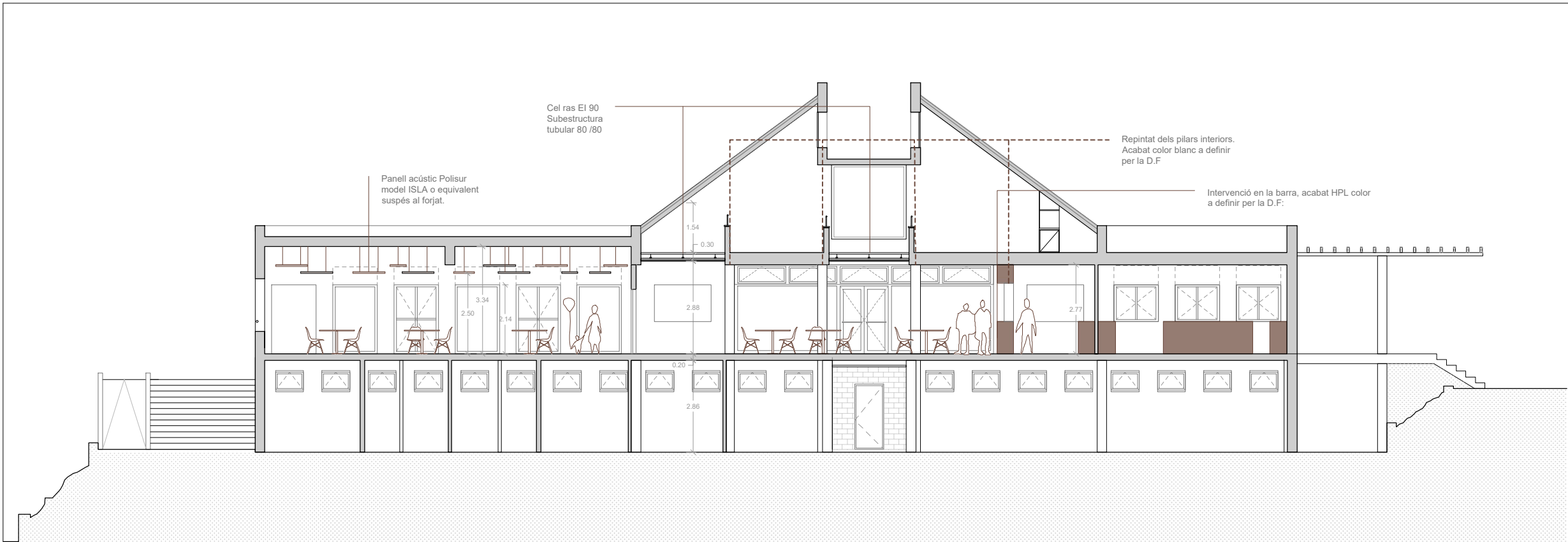
SECCIÓ 3
