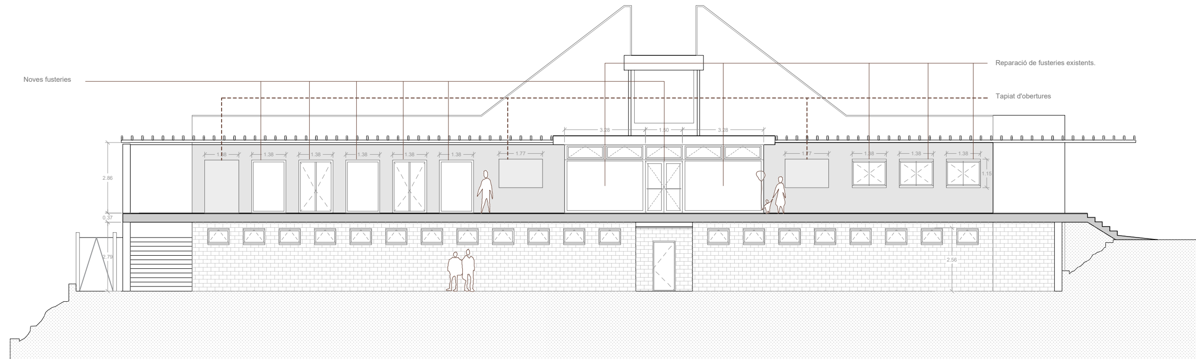
SECCIÓ 2
