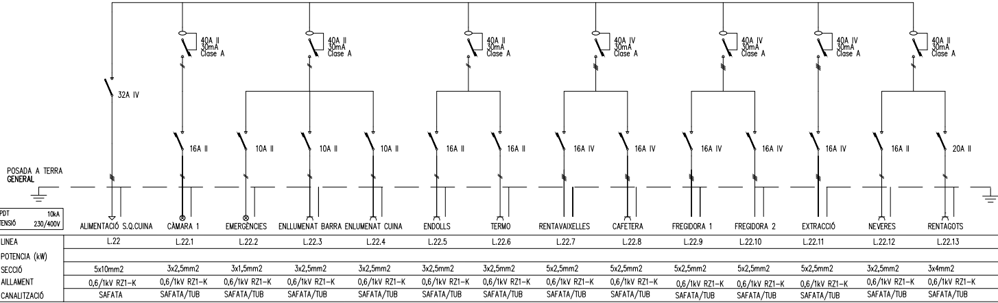
SUB-QUADRE CUINA
