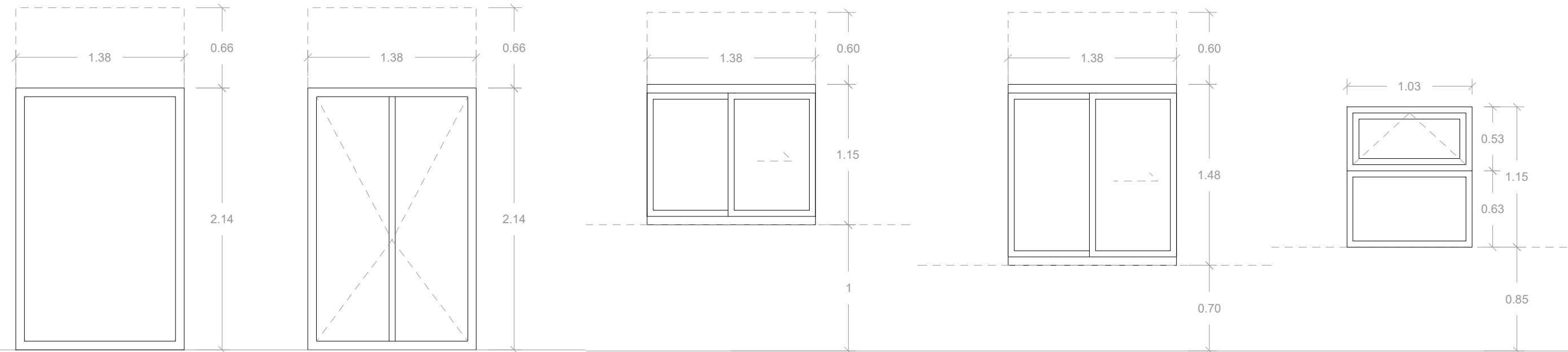
V1 BALCONERA FIXA EXTERIOR
