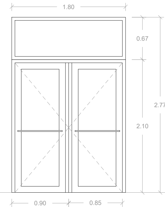
V8 PORTA SECUNDARIA V8
