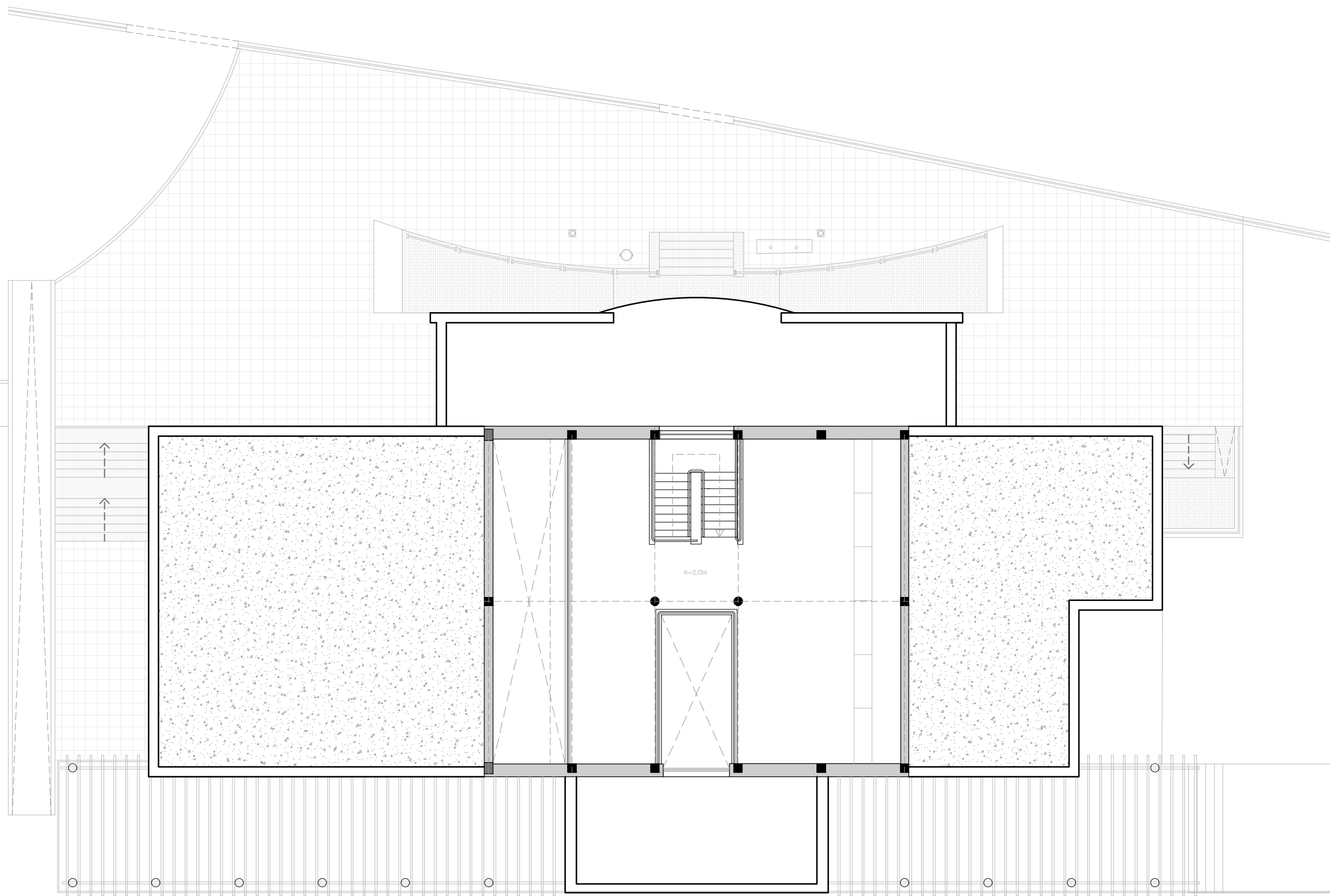
PLANTA PRIMERA | N01
