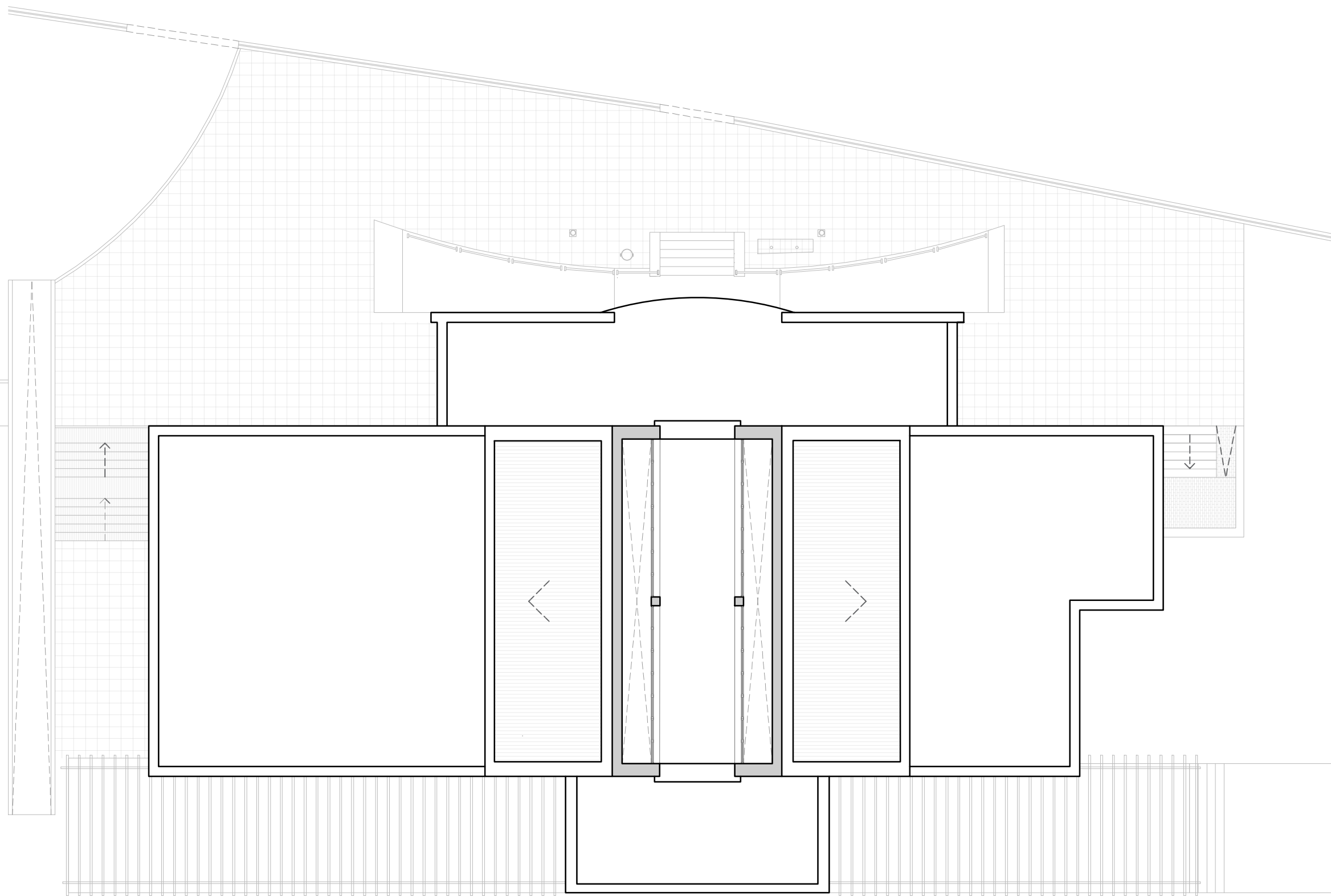
PLANTA SOTACOBERTA | N02
