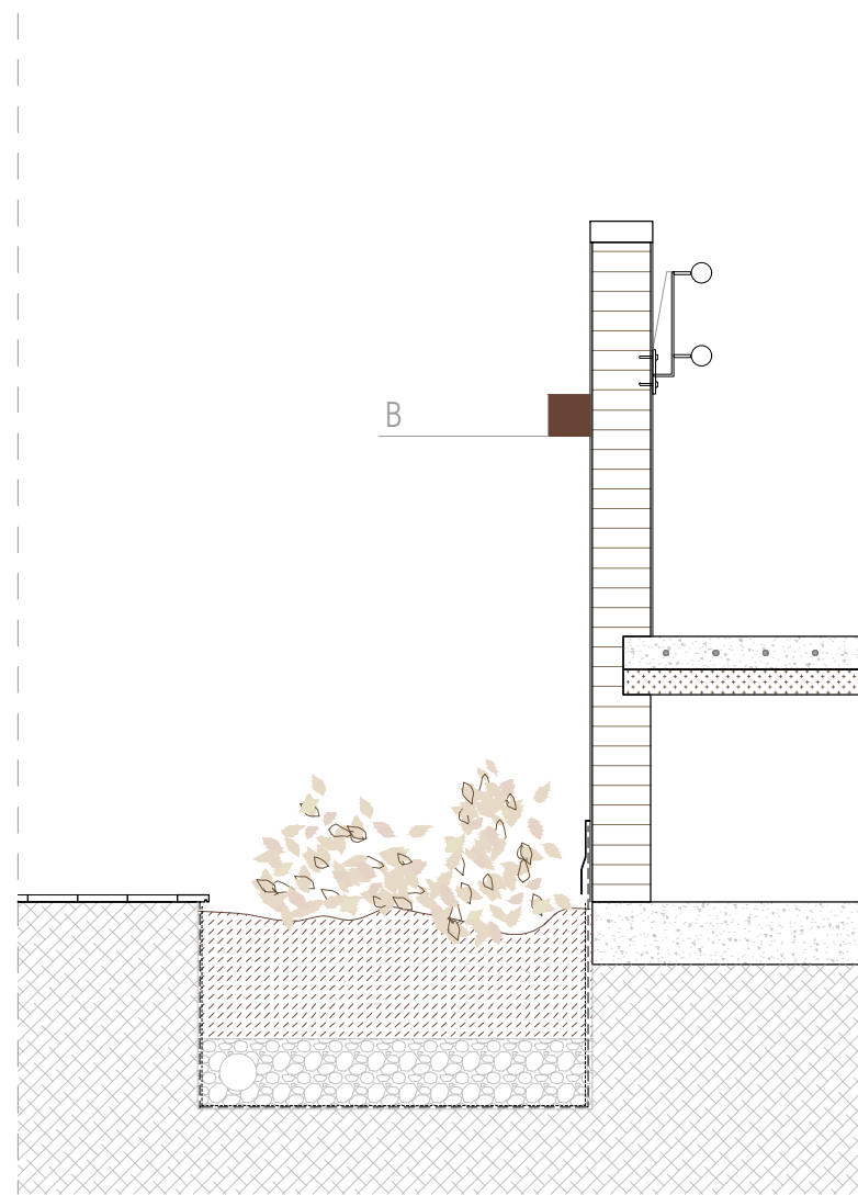
B.II.luminació de paret exterior LED d'alumini negre de dimensions 10x10x10cm. Possibilitat de tenir doble il·luminació o simple
