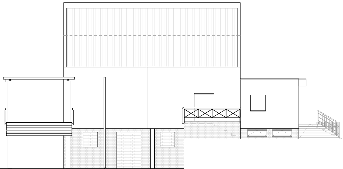
ALÇAT D
