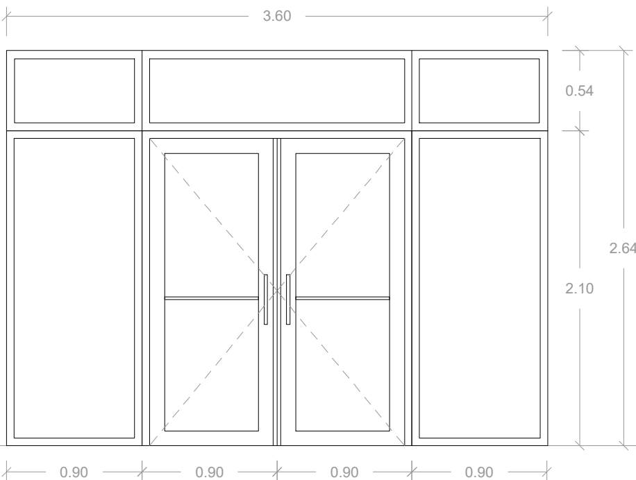
V7 CONJUNT D'ENTRADA V7
