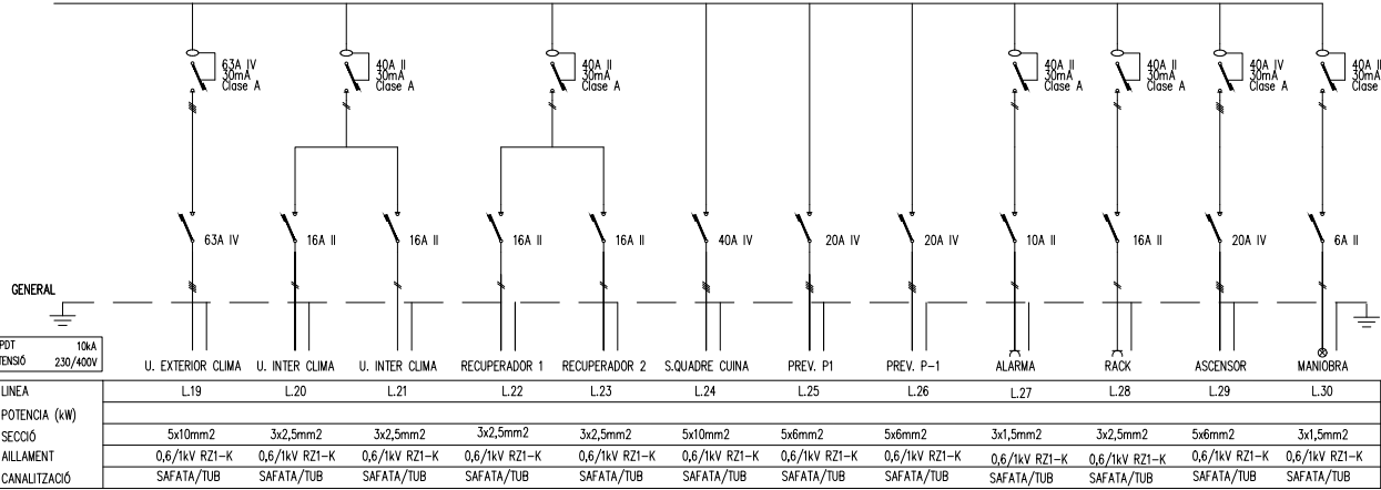
QUADRE GENERAL DE DISTRIBUCIÓ 2
