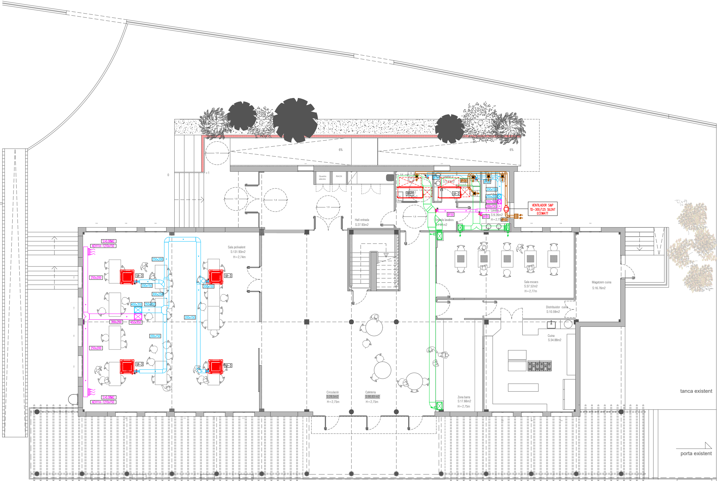
PLANTA BAIXA | N00
