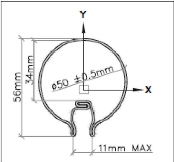
DETALL COLUMNA
