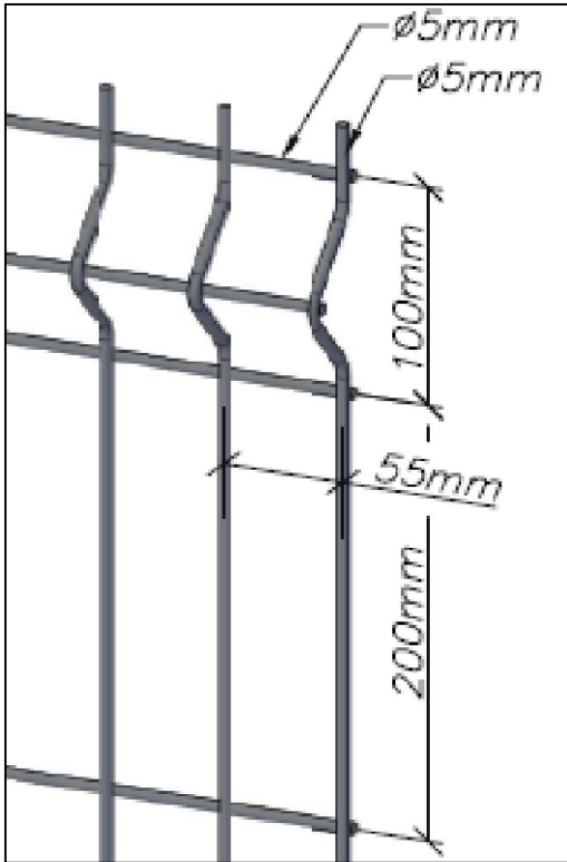
DETALL BASTIDOR
