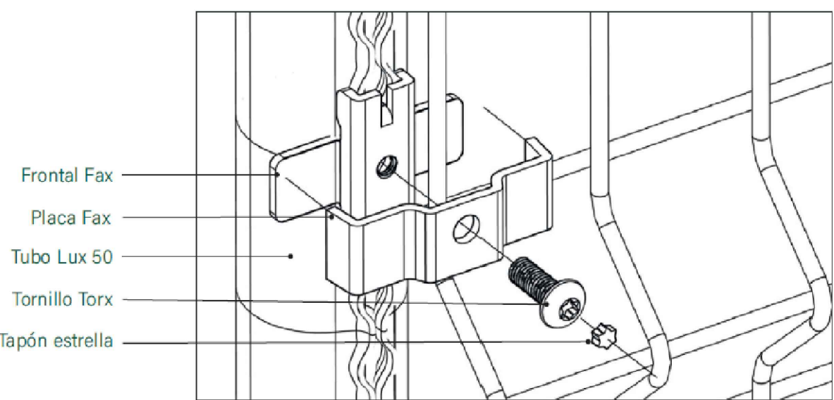
ESQUEMA D'INSTAL·LACIÓ DE LA NOVA REIXA
