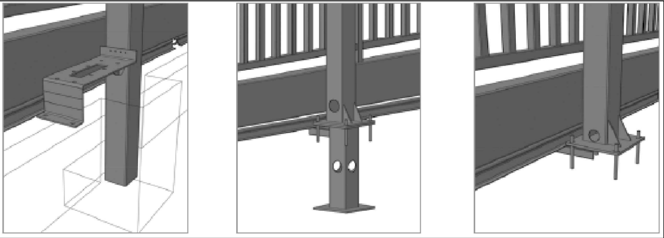
ESQUEMA SISTEMA D'ANCORATGE
