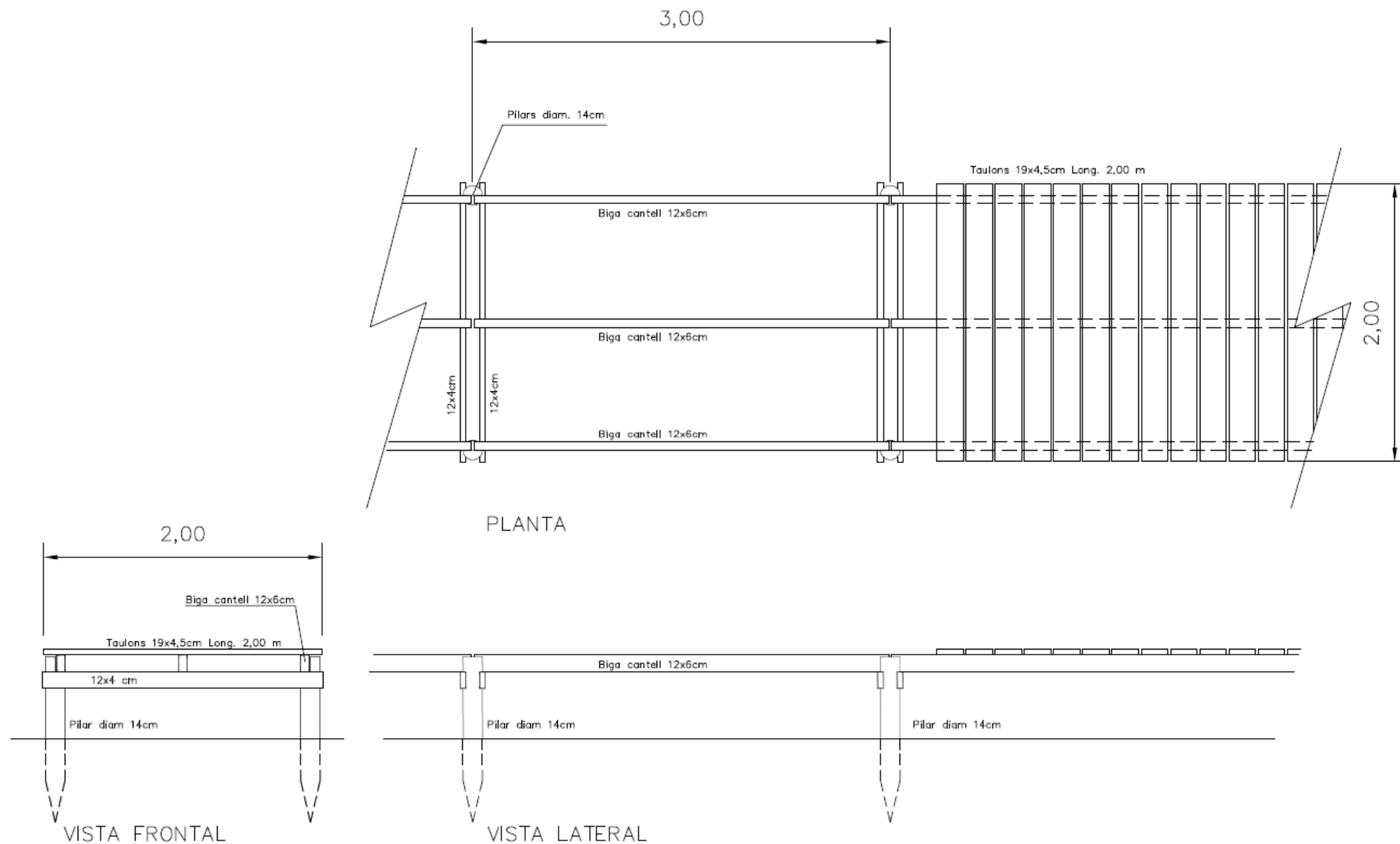
Fig. 9: Esquema constructiu de la passera
