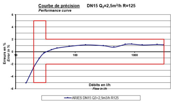
Curva de precisión Aries DN15 R125 según Directiva 2014/32/UE
