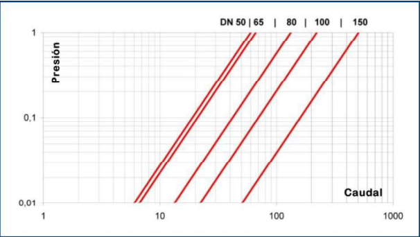
Curva de pérdida de presión
