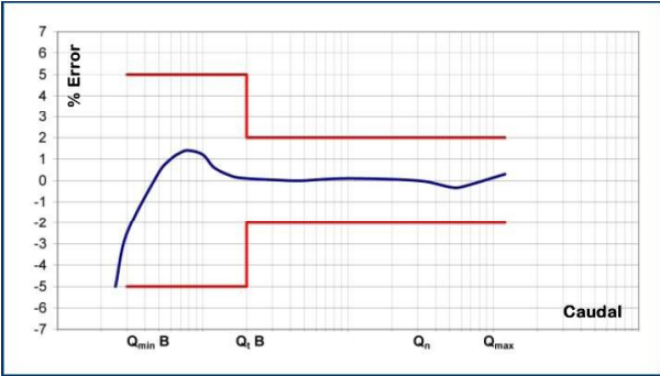
Curva característica de errores
