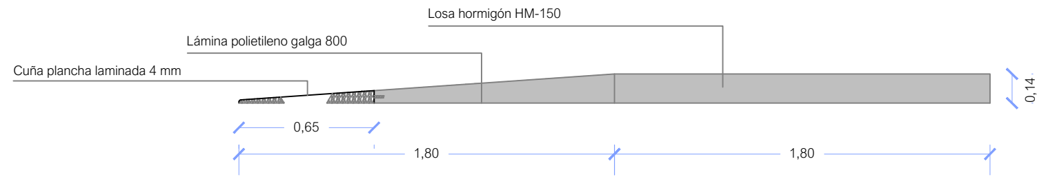
Detalle plataforma provisional acceso personas con movilidad reducida (E:1/25)
