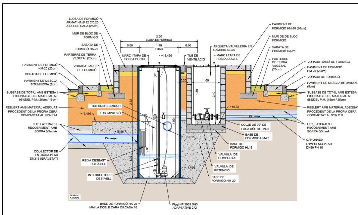
Figura 5. Detalls de la EBAR
