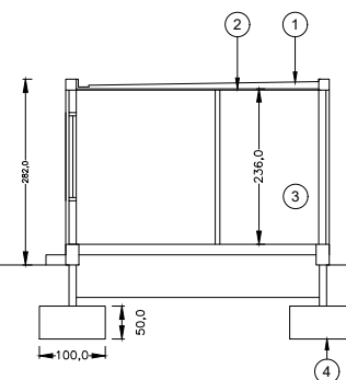
SECCIÓ A-A
