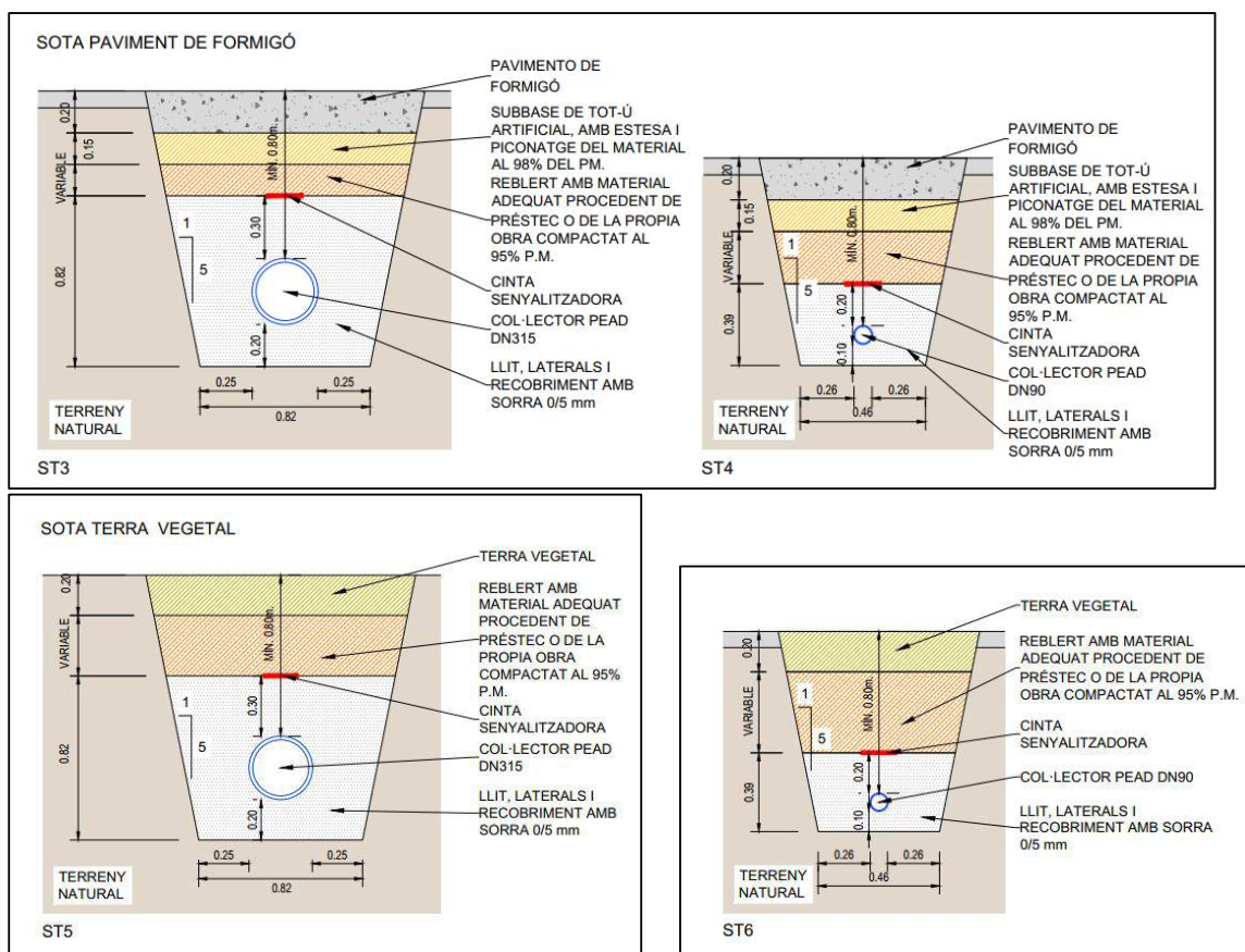
Figura 4. Seccions tipus dels col·lectors i el tub d'impulsió.
