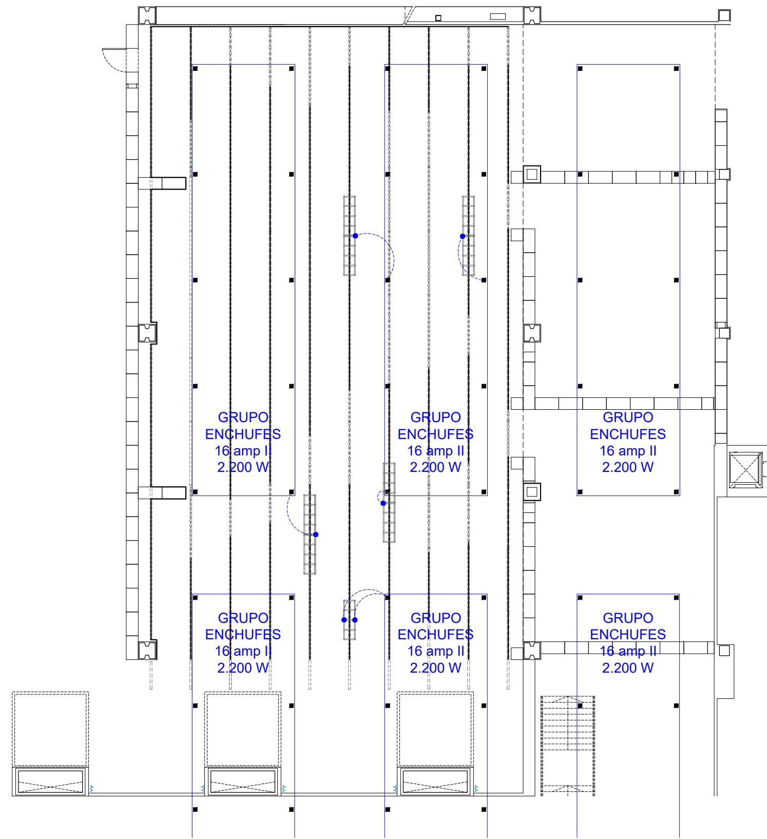
ELECTRICIDAD: SUELO PLANTA
