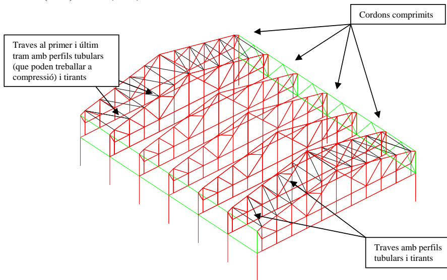
figura 8 – Esquema noves de triangulacions en mòdul entre junts de 7 encavallades (tram façana oest-junt)
