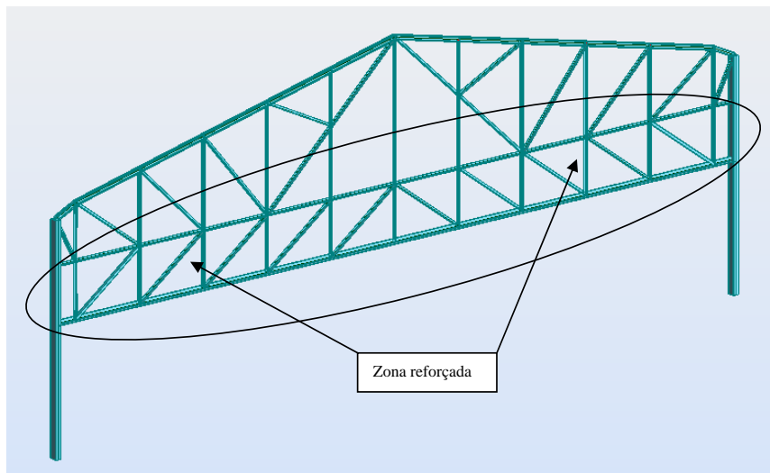
figura 10 – Detall pòrtic tipus reforçat (programa ROBOT MILLENIUM)
