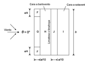
(b) Direcció del vent \theta = 0^\circ
