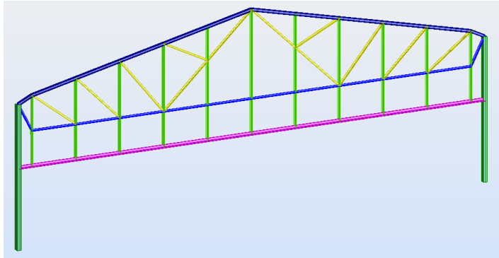
figura 7 – detall pòrtic tipus programa ROBOT MILLENIUM
