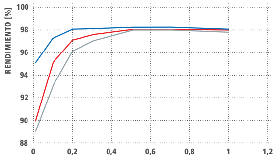
POTENCIA DE SALIDA ESTANDARIZADA P_{dc}/P_{dcr} ■ 580 V dc ■ 800 V dc ■ 930 V dc
