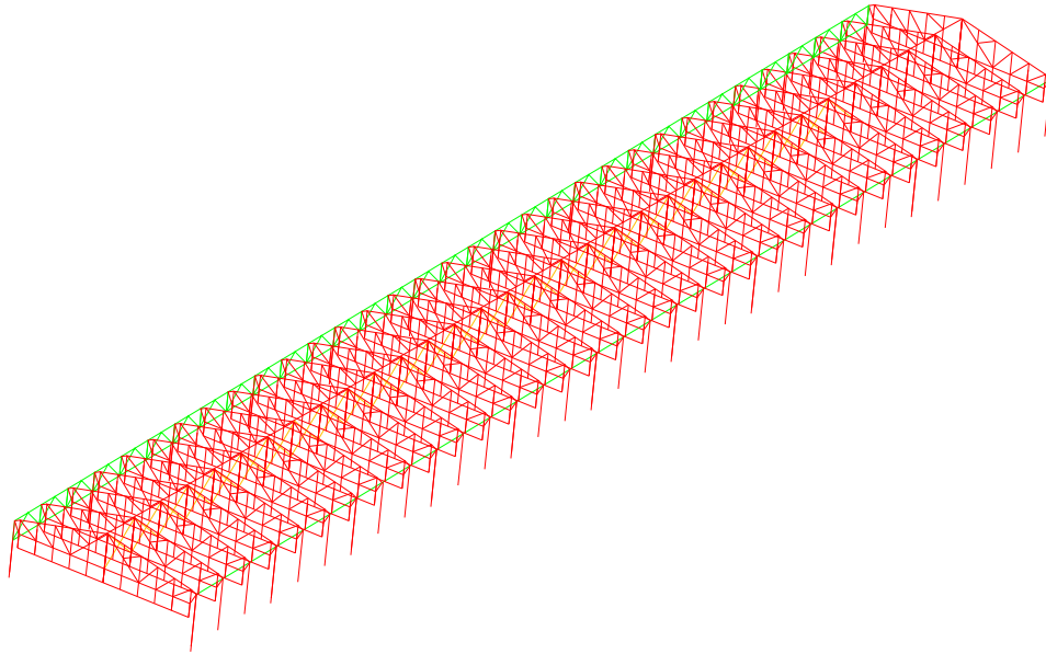
figura 5 – Esquema nau sencera
