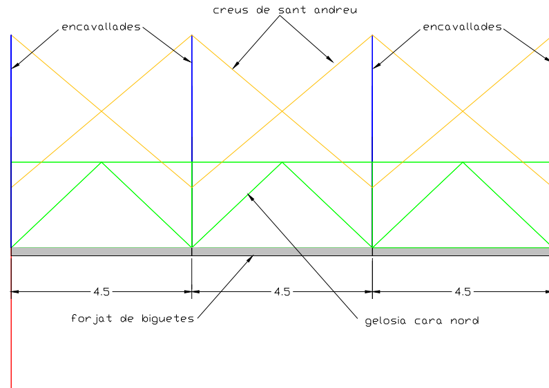
figura 3 – Detall alçat gelosia
