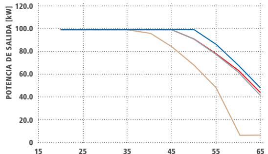
TEMPERATURA AMBIENTE [°C] ■ 580 V dc ■ 800 V dc ■ 850 V dc ■ 930 V dc
