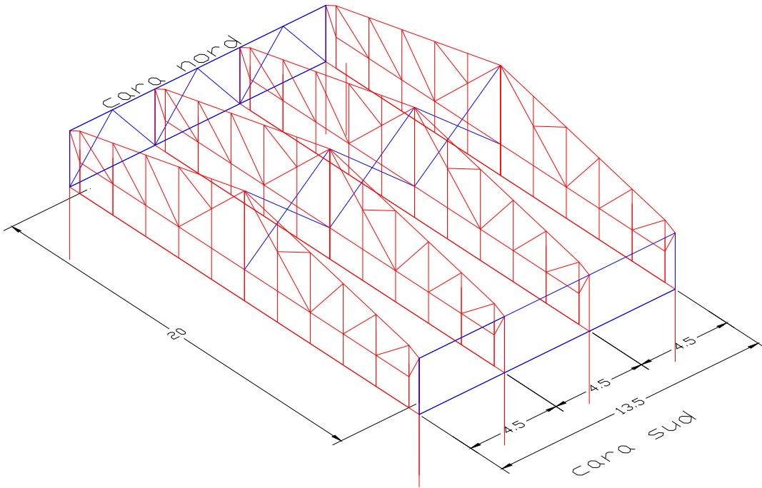
figura 2 – Esquema d'estructura de coberta
