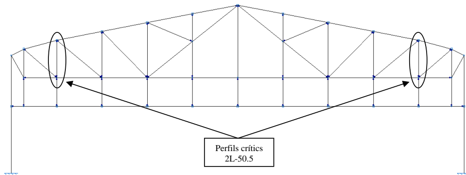
figura 6 – detall pòrtic tipus programa METAL 3D
