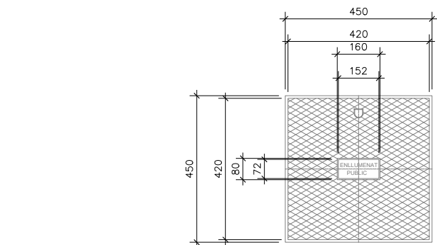
TAPA I MARC (TRONETA 0.45x0.45)
