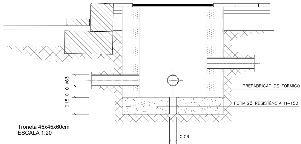
TAPA I MARC (TRONETA 0.45x0.45)
