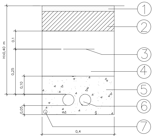
Rasa tipus per a entubar cables a zona creuament vials ESCALA 1:10
