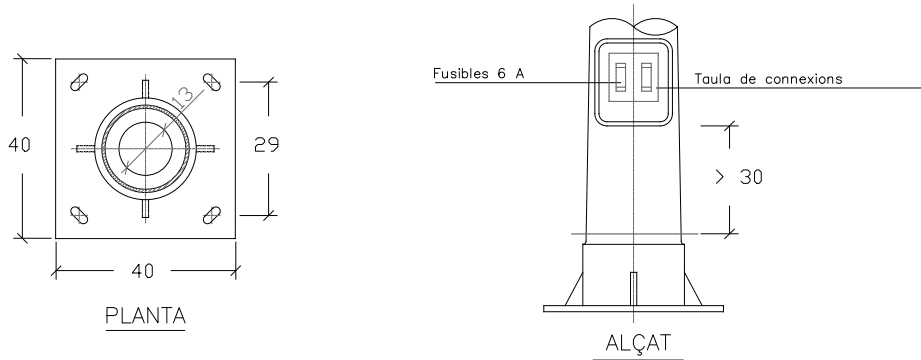
ANCORATGE DE LES COLUMNES I BACULS
