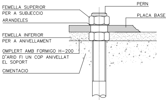
DETALL I FONAMENT COLUMNA TIPUS I PRESA DE TERRA
