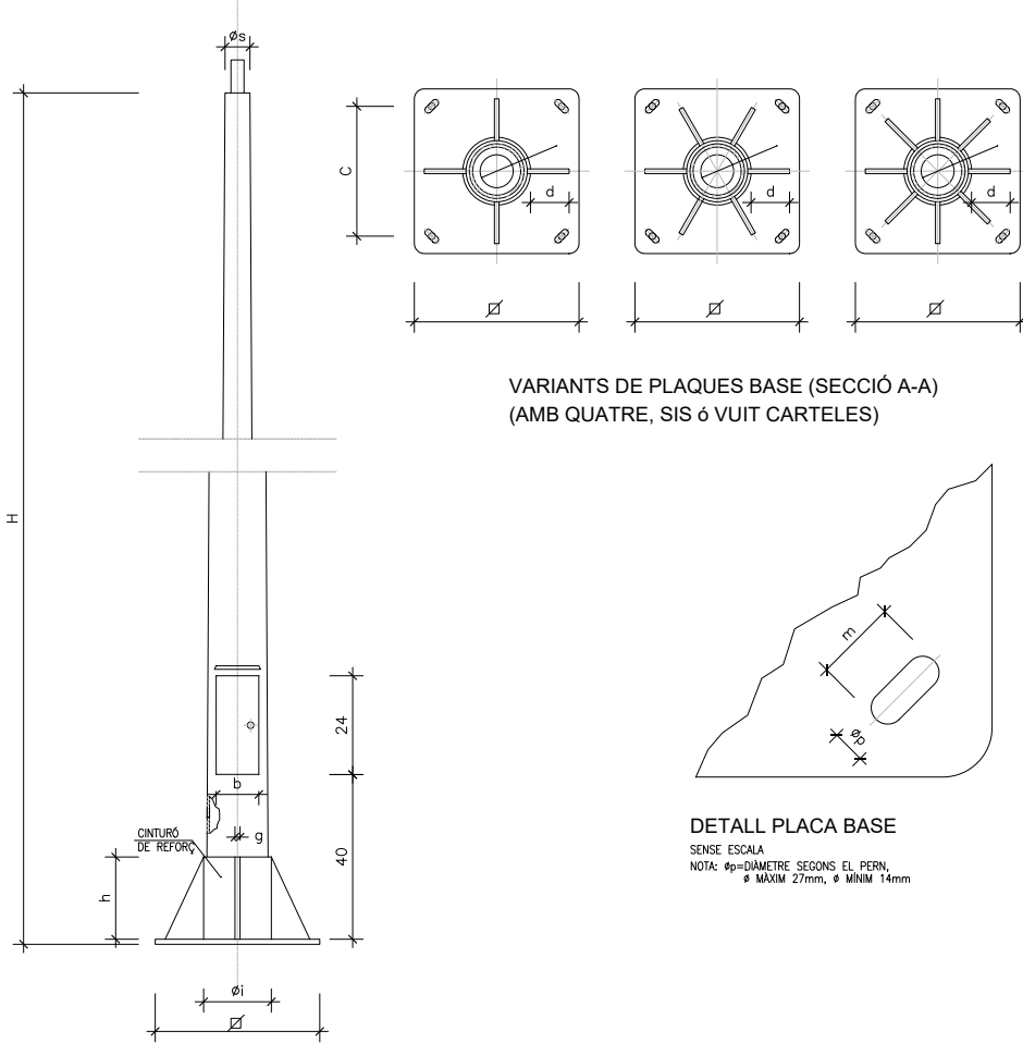
QUADRES I DETALLS D'ALÇADES I DIMENSIONATS TOTES LES ALÇADES EN METRES . TOTS ELS DIMENSIONATS EN MIL·LÍMETRES
