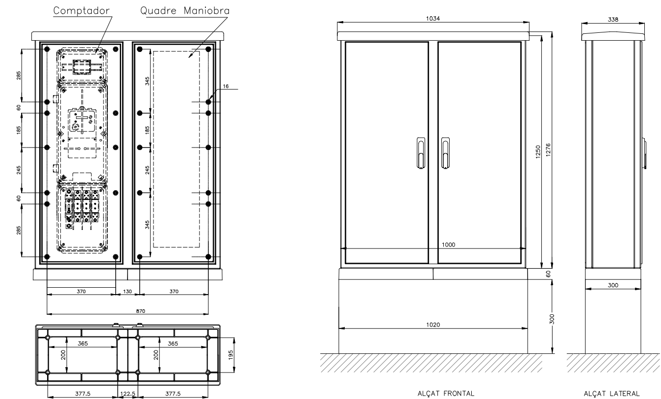
DIMENSIONS I DISTRIBUCIO APARELLATGE QUADRE CAHORS O SIMILAR
