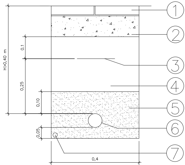
Rasa tipus per a entubar cables a zona de voreres ESCALA 1:10
