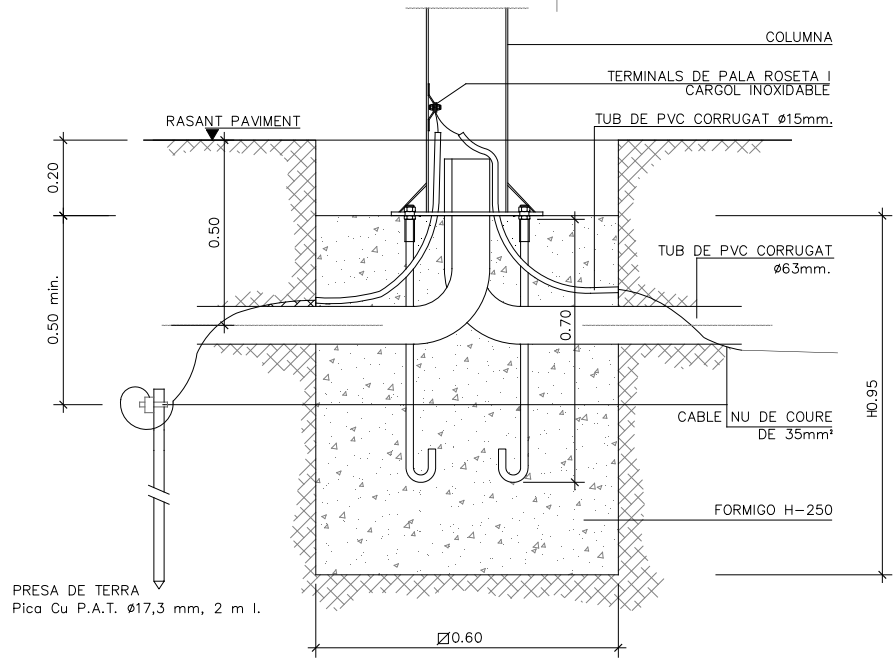
DETALL I FONAMENT COLUMNA TIPUS I PRESA DE TERRA
