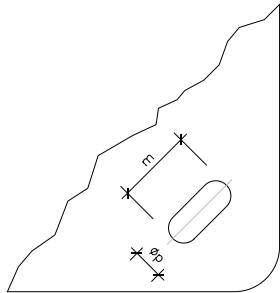
DETALL PLACA BASE SENSE ESCALA NOTA: Øp=DIÀMETRE SEGONS EL PERN. Ø MAXIM 27mm, Ø MINIM 14mm
