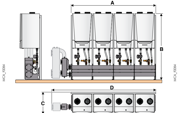
Alineación en el suelo de cuatro calderas
