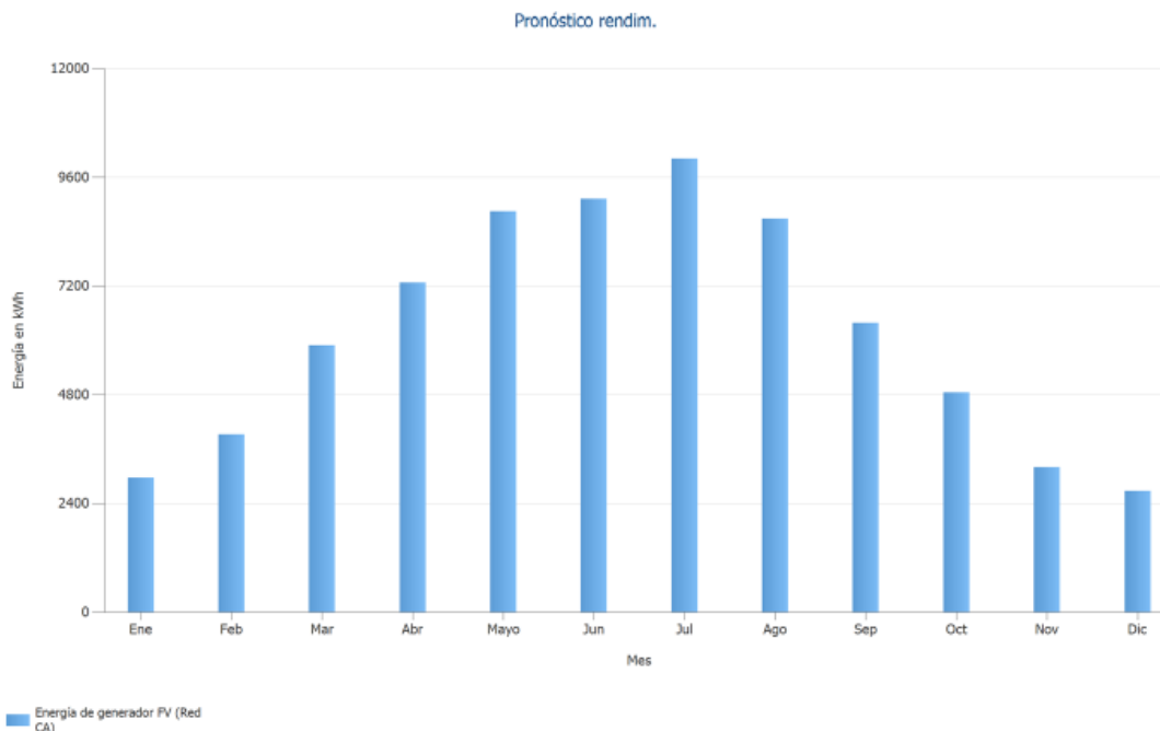
Figura 10- Gràfica de generació elèctrica anual. FONT: PVsol
