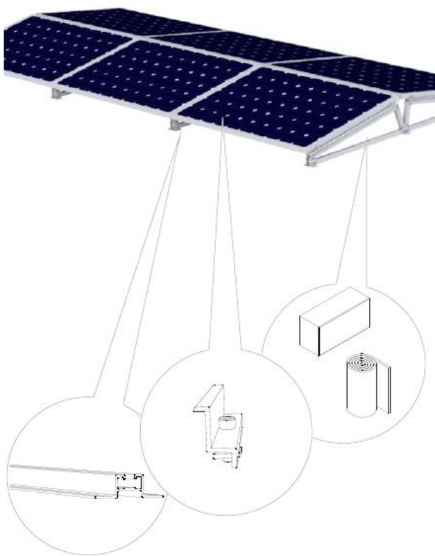
Figura 7. Estructura bi-orientada E-O. Font: Solarstem
