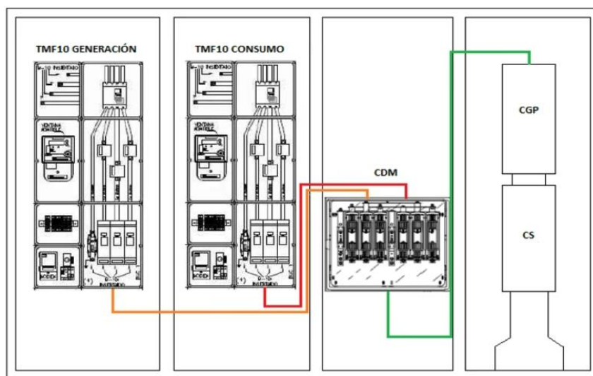
Figura 10 Esquema de connexió d'instal·lacions receptores per instal·lacions d'autoconsum col·lectiu o de diferents titulars. Font: E-distribución
