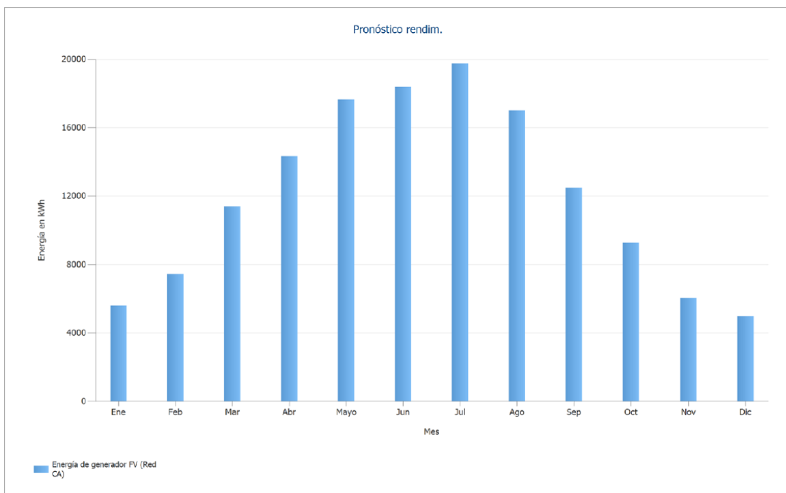
Figura 9. Generació fotovoltaica anual
