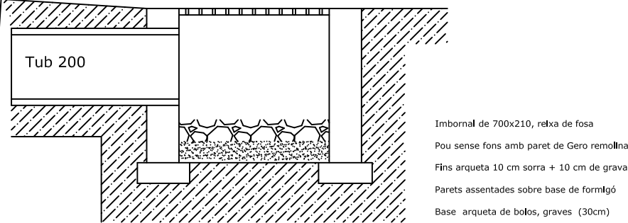
Detall Arqueta Sortida
