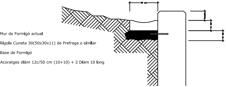
Detall Canal de Formigó
