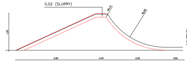
Detalle Perfil Peraltes
