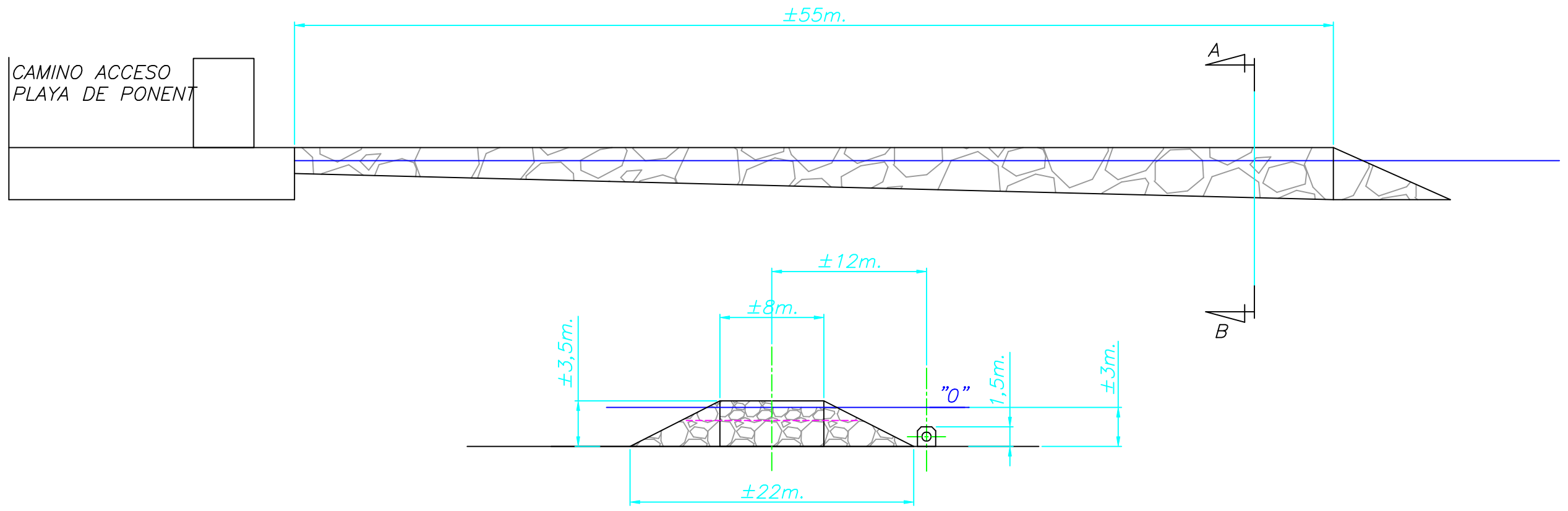
SECCION A-B
