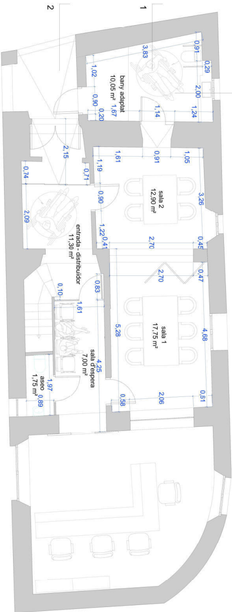
PLANTA 1/75
