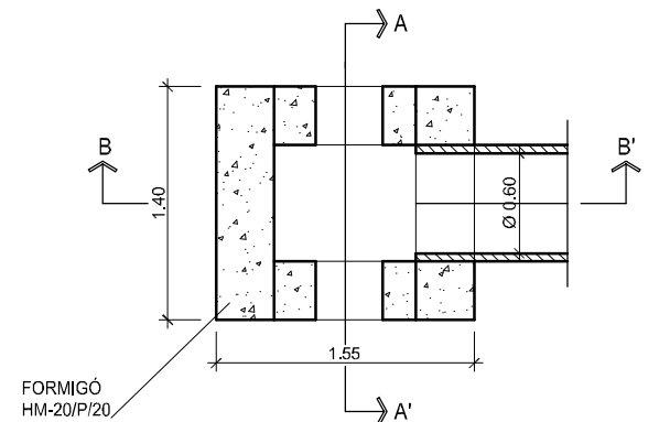
PLANTA (SECCIÓ C-C')
