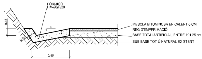
DETALLS CUNETA ESCALA 1/50
