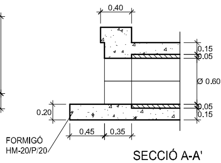
DETALL DESEMBOCADURA ESCALA 1/50
