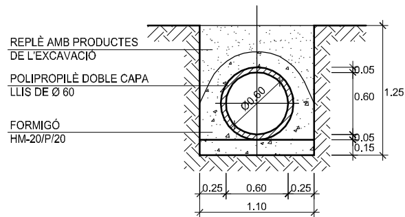
DETALL SECCIONS RASES ESCALA 1/50
