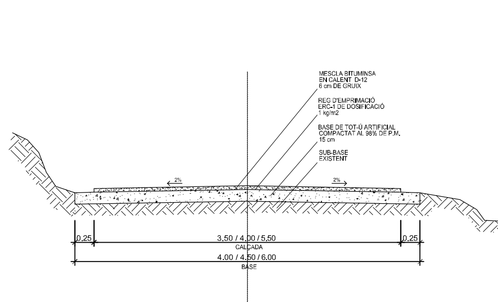
SECCIÓ TIPUS CAMI ESCALA 1/50
