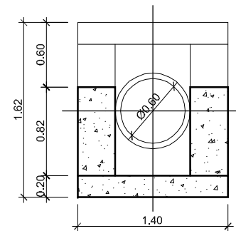
SECCIÓ A-A'
