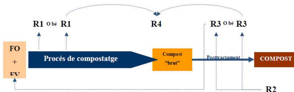
Diagrama de flux amb la ubicació dels rebutjos de les plantes
