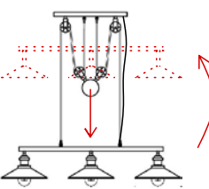
Esquema politja per elevar làmpades sobre billar
