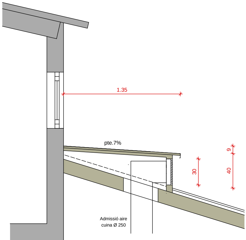
Secció
