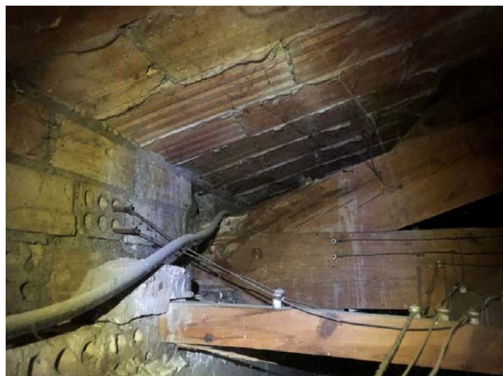
Imatge 12: Recolzament d'encavallada núm. 2 sobre de l'espai del menjador. La paret de l'esquerra de la imatge correspon a la paret entre el menjador i la cuina. Marques d'humitat a la part superior a la trobada entre el tirant inferior i l'element coplanar a la vessant.
