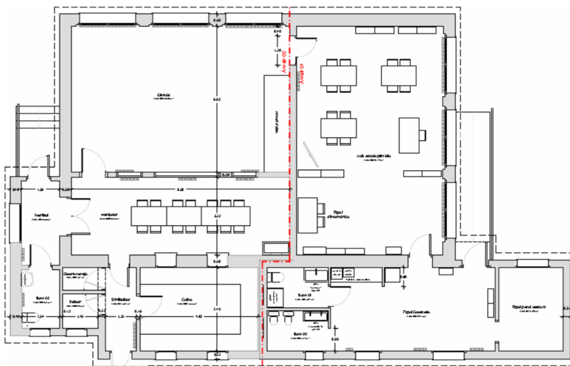
Imatge 03: Planta de l'immoble amb els dos àmbits definits. Àmbit 01 al costat dret amb les dependències que requereixen actuacions per habilitar el 1er cicle d'educació infantil i l'Àmbit 02 a l'esquerra amb la resta de dependències i a on es completen les actuacions de fals sostre i coberta.
