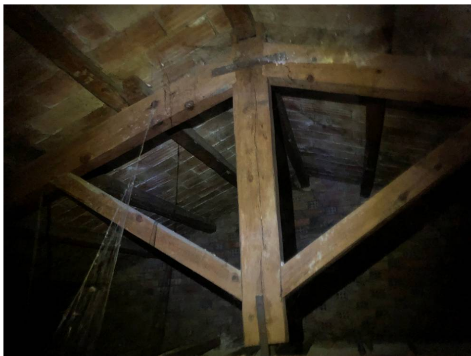
Imatge 06: Part central de l'encavallada nord que sostenta la coberta amb corretges i tauler d'encadellat ceràmic.
