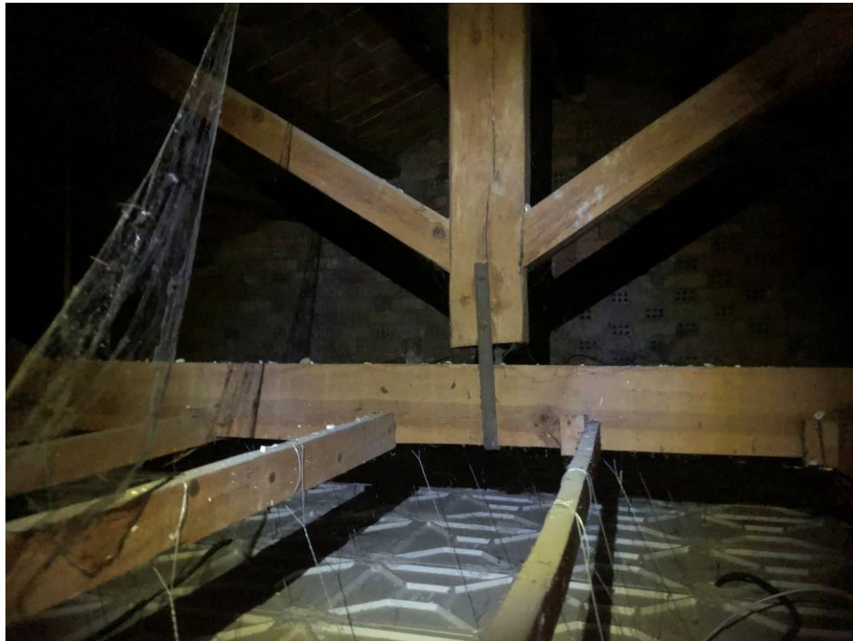
Imatge 07: Part central inferior de l'encavallada nord amb la subestructura de sosteniment del fals sostre.
