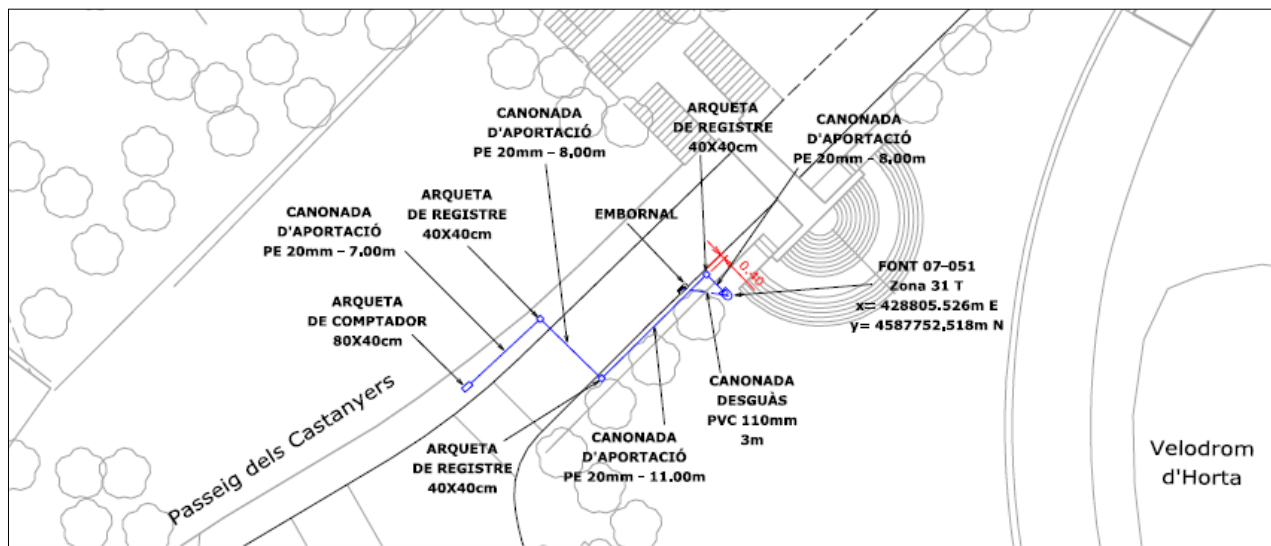
Figura 1. Exemple segregació font de beure
