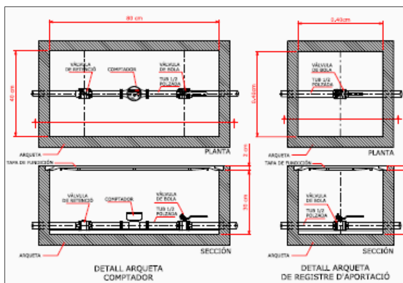
Figura 2. Exemple arqueta font de beure
