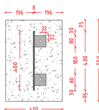
ANCORATGE PEU COR-TEN Escala 1:10
