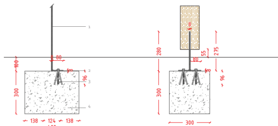
ANCORATGE PEU COR-TEN Escala 1:10
