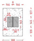
ANCORATGE PEU FUSTA (140x140 mm) Escala 1:10
