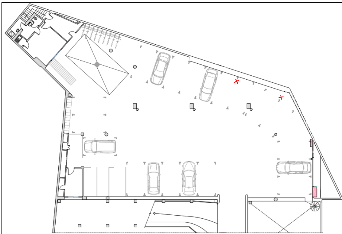
Figura 6. Ubicació de les futures estacions de recarrega de vehicle elèctric (X) en la planta 0.
