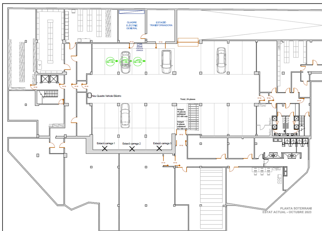
Figura 3. Ubicació del sub quadre de vehicle elèctric (□) i estacions de recarrega de vehicle elèctric doble(x).
