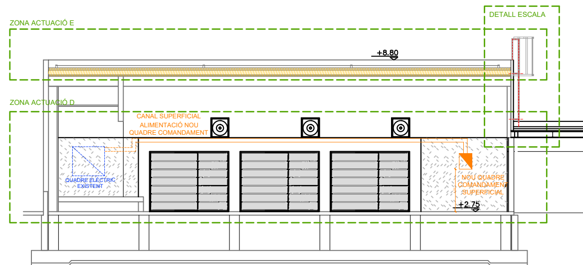
SECCIÓ AA' GIMNÀS
