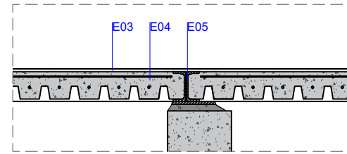
DETALL CONSTRUCTIU FORJAT COL-LABORANT EXISTENT
