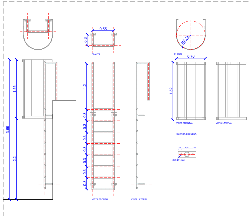
DETALL ESCALA ACCÉS COBERTA
