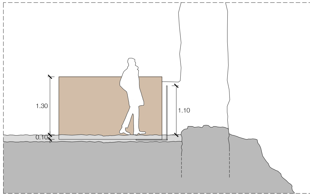
SECCIÓ
