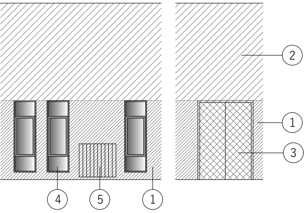
ALÇAT INTERIOR TIPUS DEL GIMNÀS:
