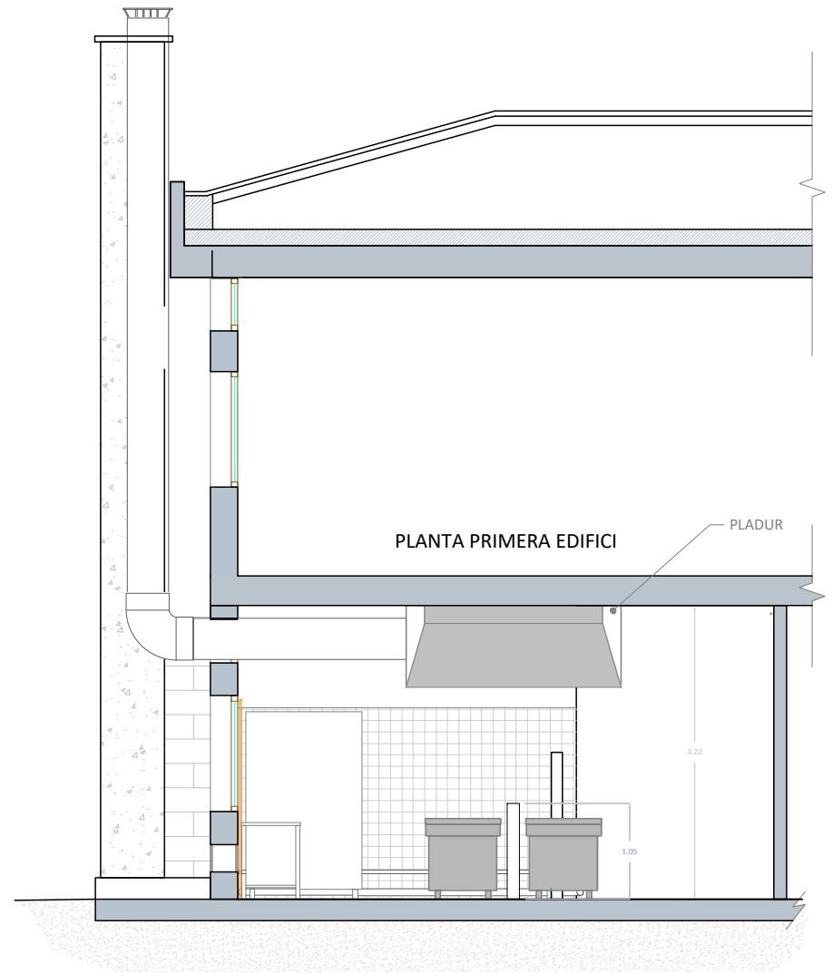
SECCIÓ C-C'
