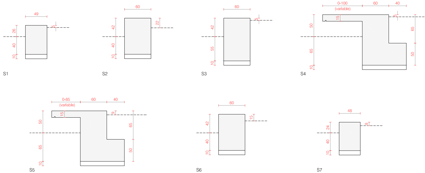
DEFINICIÓ GEOMÈTRICA MUR DE FORMIGÓ. SECCIONS E: 1/50
