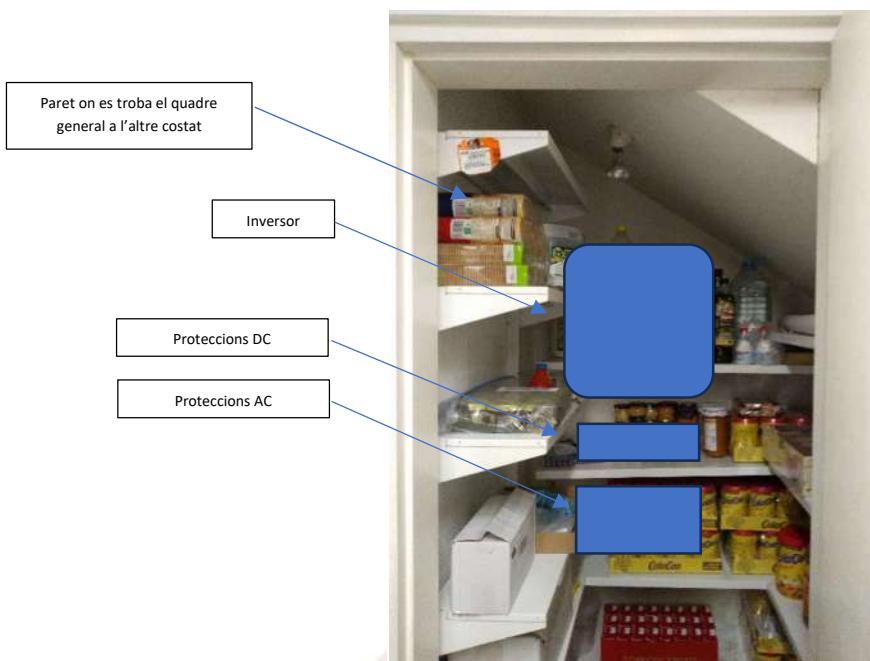
Figura 10. Sala per a l'inversor i els quadres de proteccions
