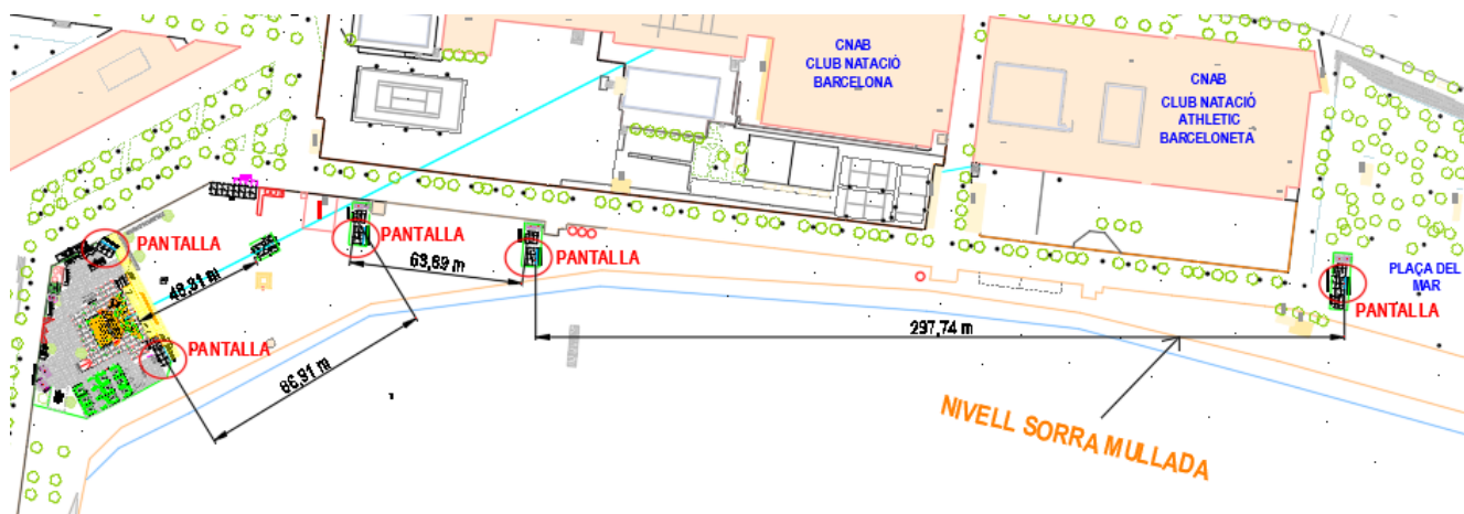
Plànol preliminar de la situació del muntatge
