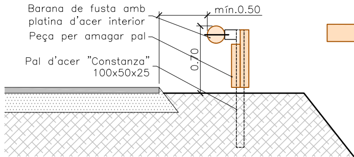
DETALL BOCA DE SORTIDA
