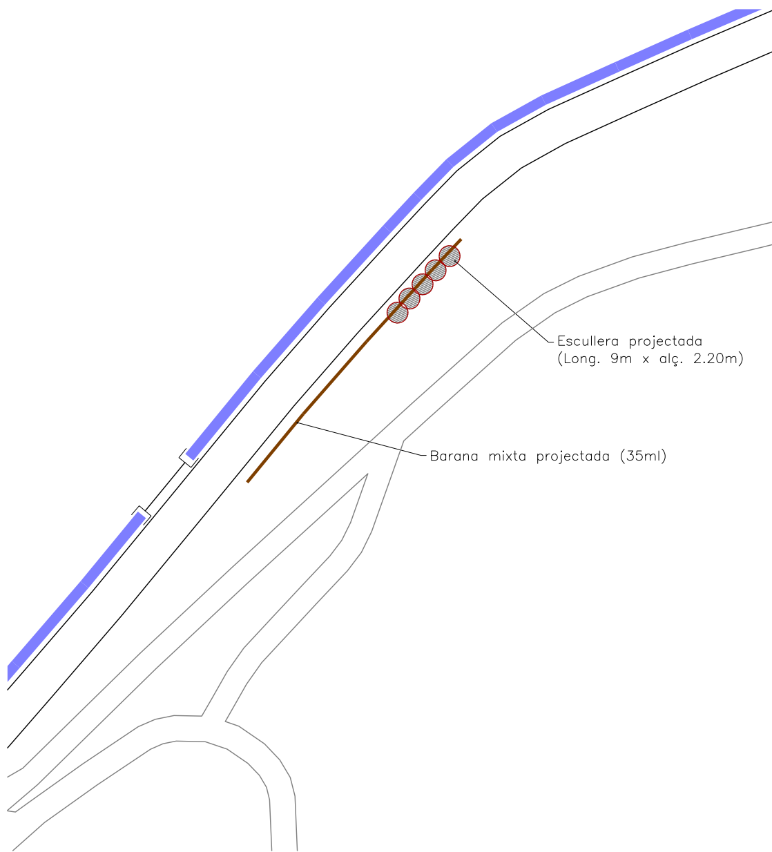
PLANTA GENERAL E: 1/500
