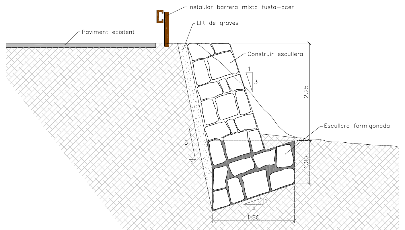
SECCIÓ TIPUS ESCULLERA E: 1/50
