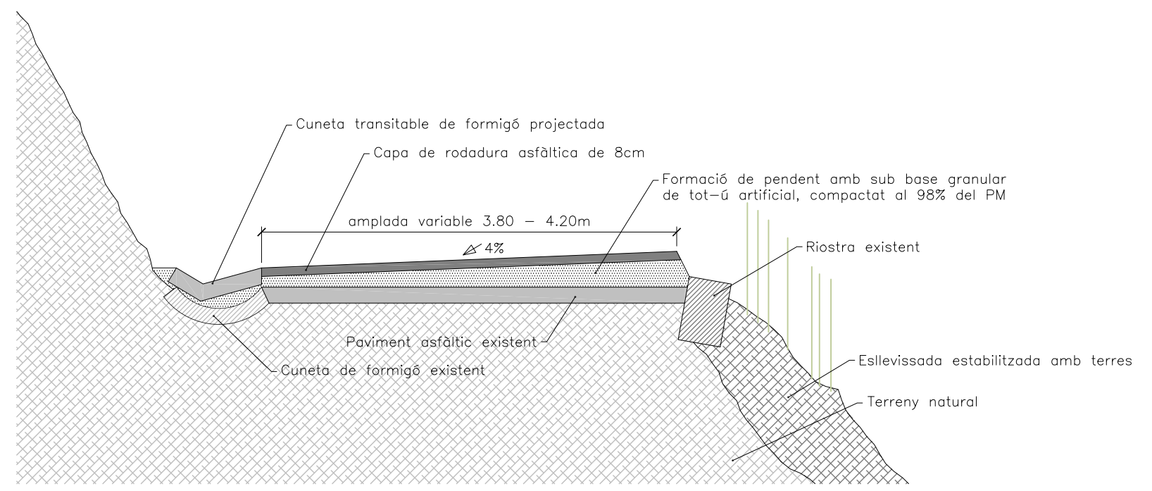
SECCIÓ TIPUS E: 1/50
