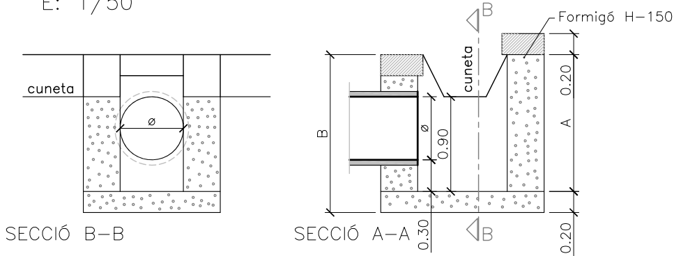
DETALL BOCA D'ENTRADA E: 1/50
