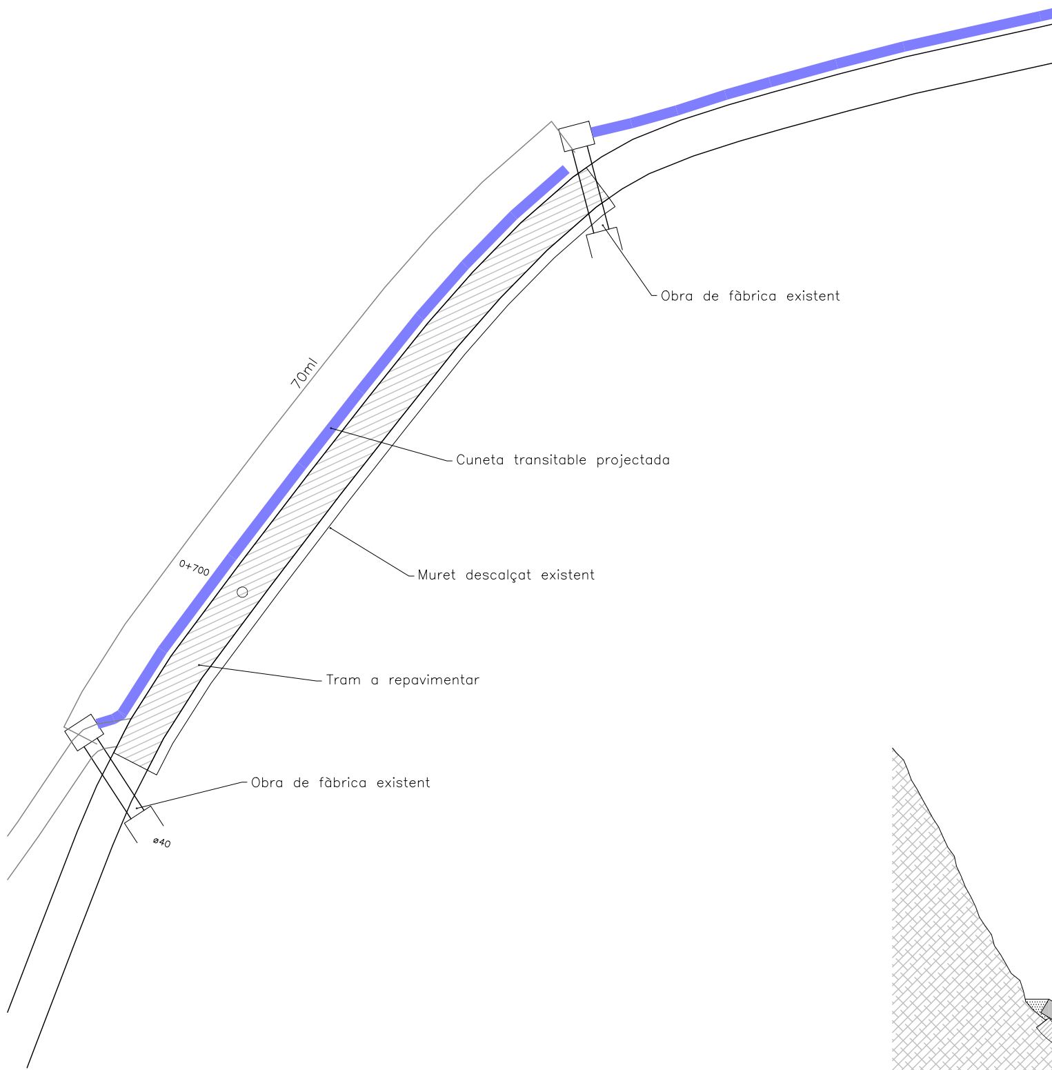
PLANTA GENERAL E: 1/500
