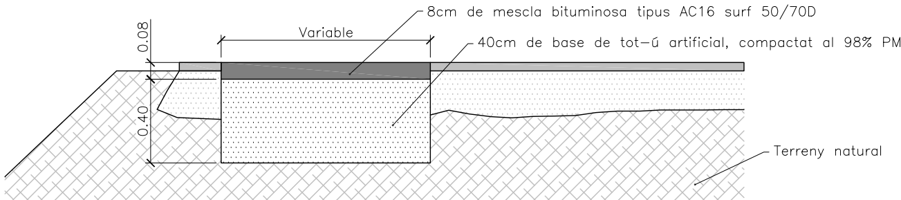
SECCIÓ TIPUS ARRANJAMENT DE FLONJALLS E: 1/25
