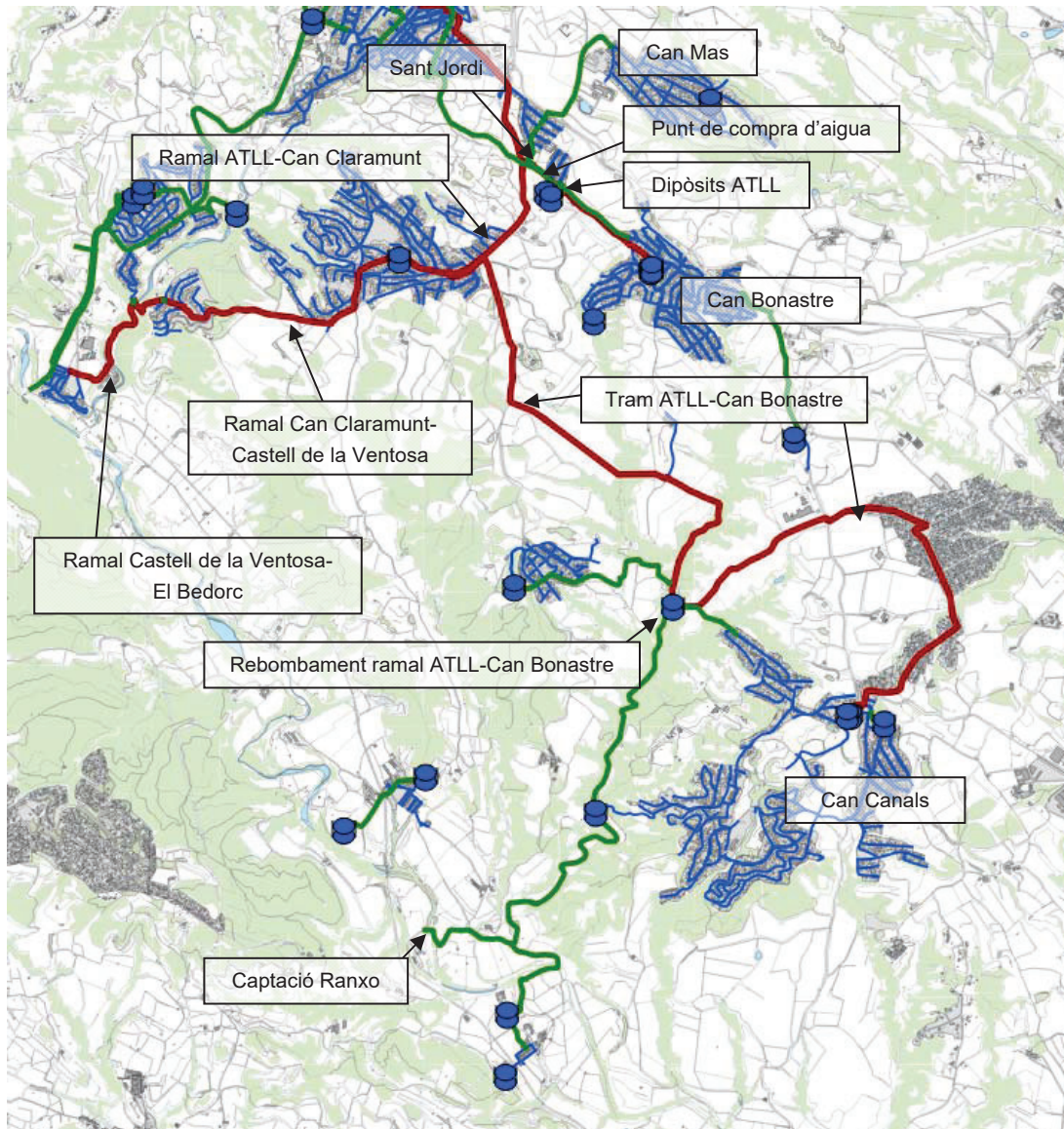
Figura 6. Planta esquemàtica del ramal ATLL-Can Bonastre Ramal ATLL-Can Claramunt, Castell de la Ventosa, el Bedorc, Can Creixell, Can Canals i la Fortesa
