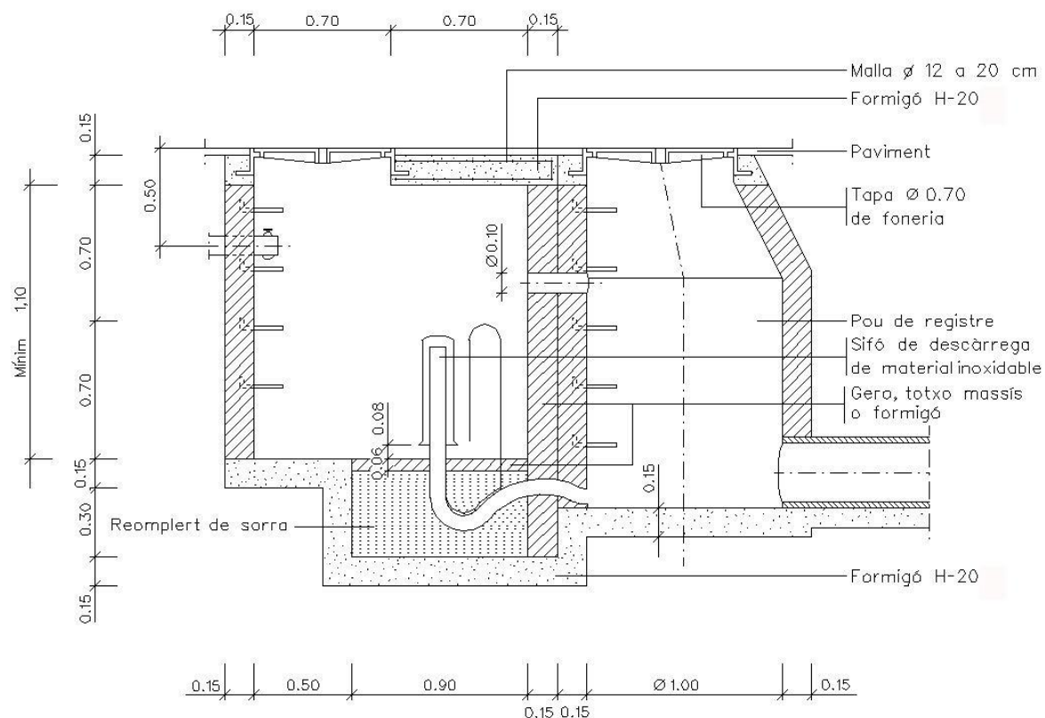
Camra de descàrrega amb pou
