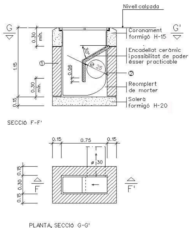
Embornalsifònic " in situ "
