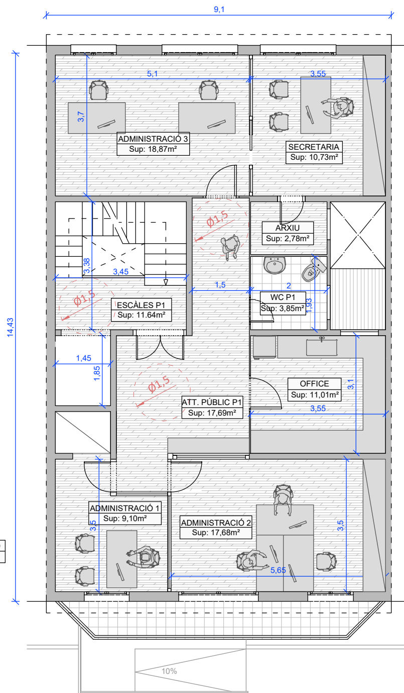
PLANTA PRIMERA Sup. construïda: 128,20 m2
