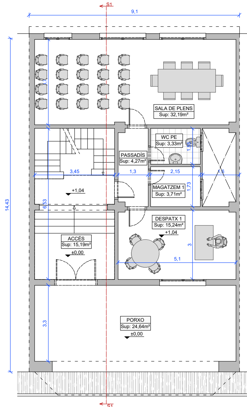
PLANTA BAIXA Sup. construïda: 128,20 m²
