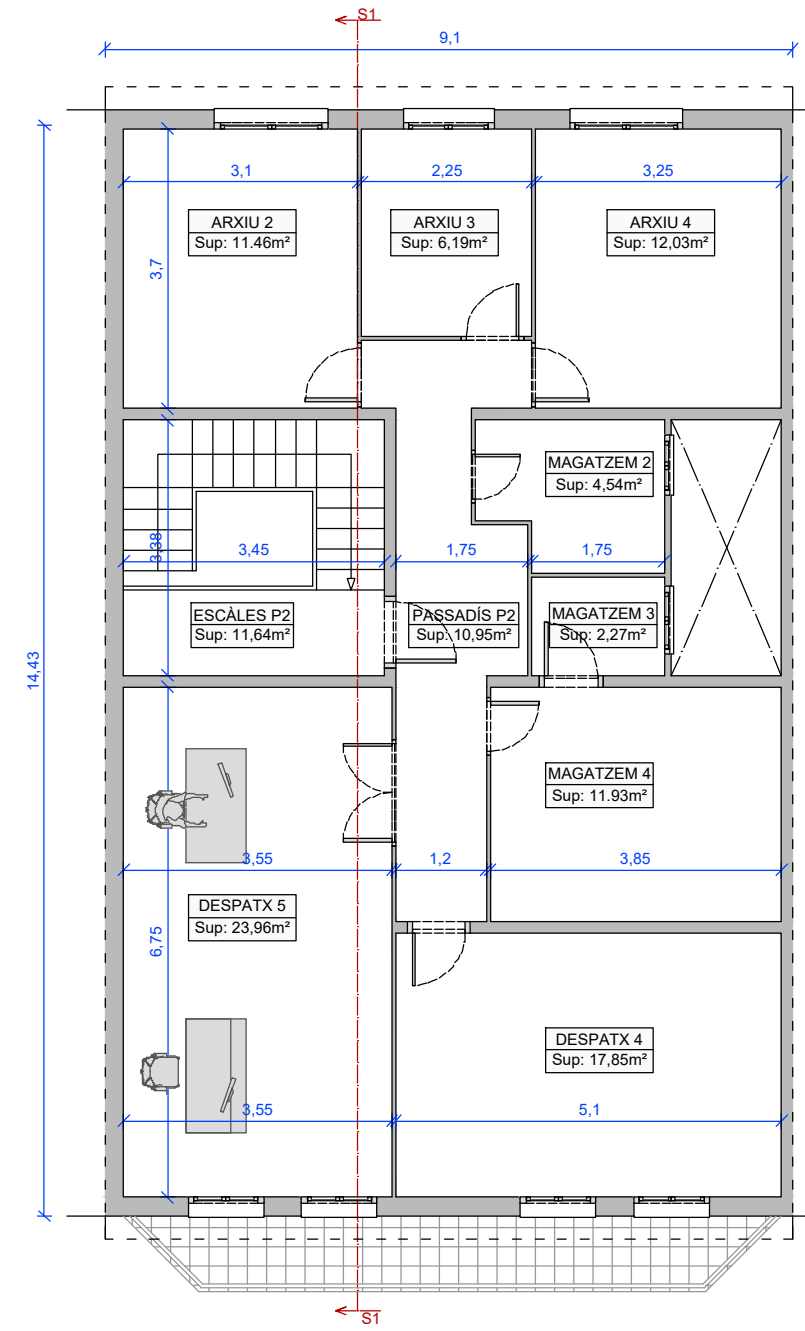
PLANTA SEGONA Sup. construïda: 128,20 m²
