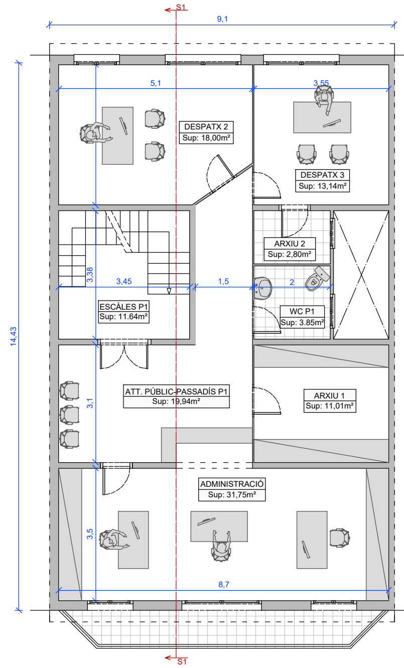
PLANTA PRIMERA Sup. construïda: 128,20 m²
