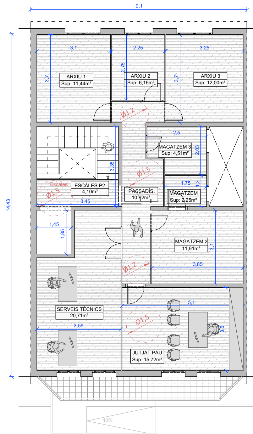
PLANTA SEGONA Sup. construïda: 128,20 m2
