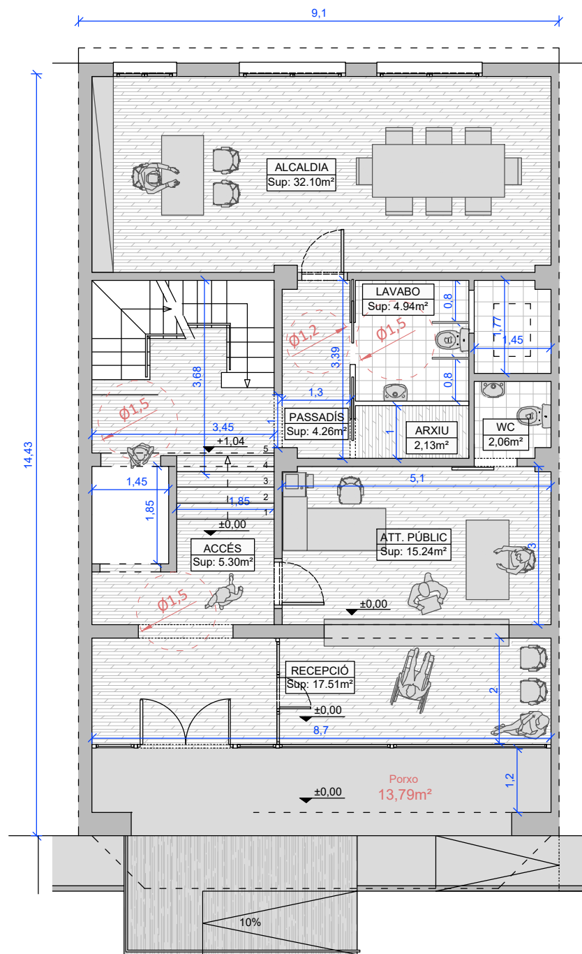
PLANTA BAIXA Sup. construïda: 128,20 m2
