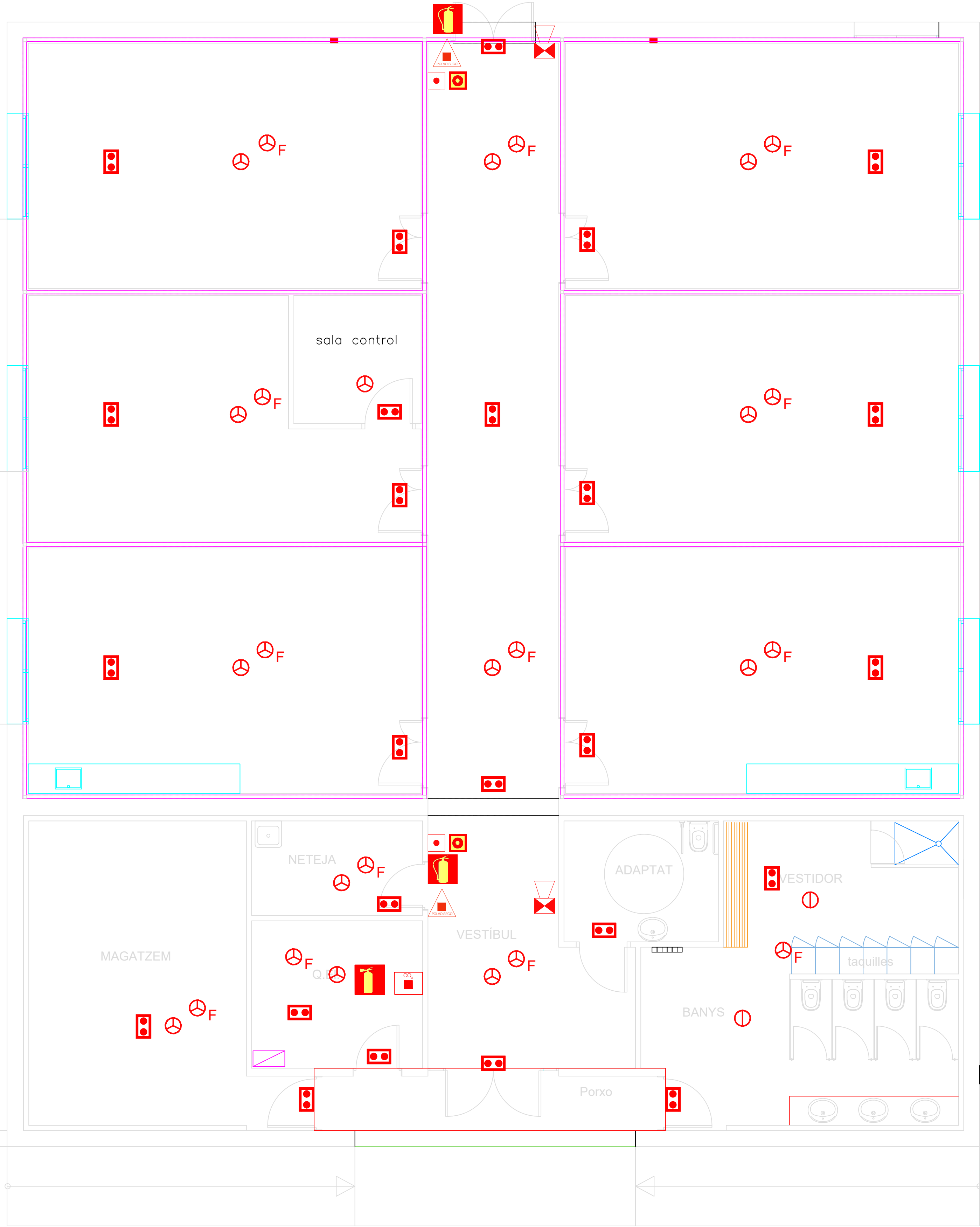
PLANTA BAIXA
