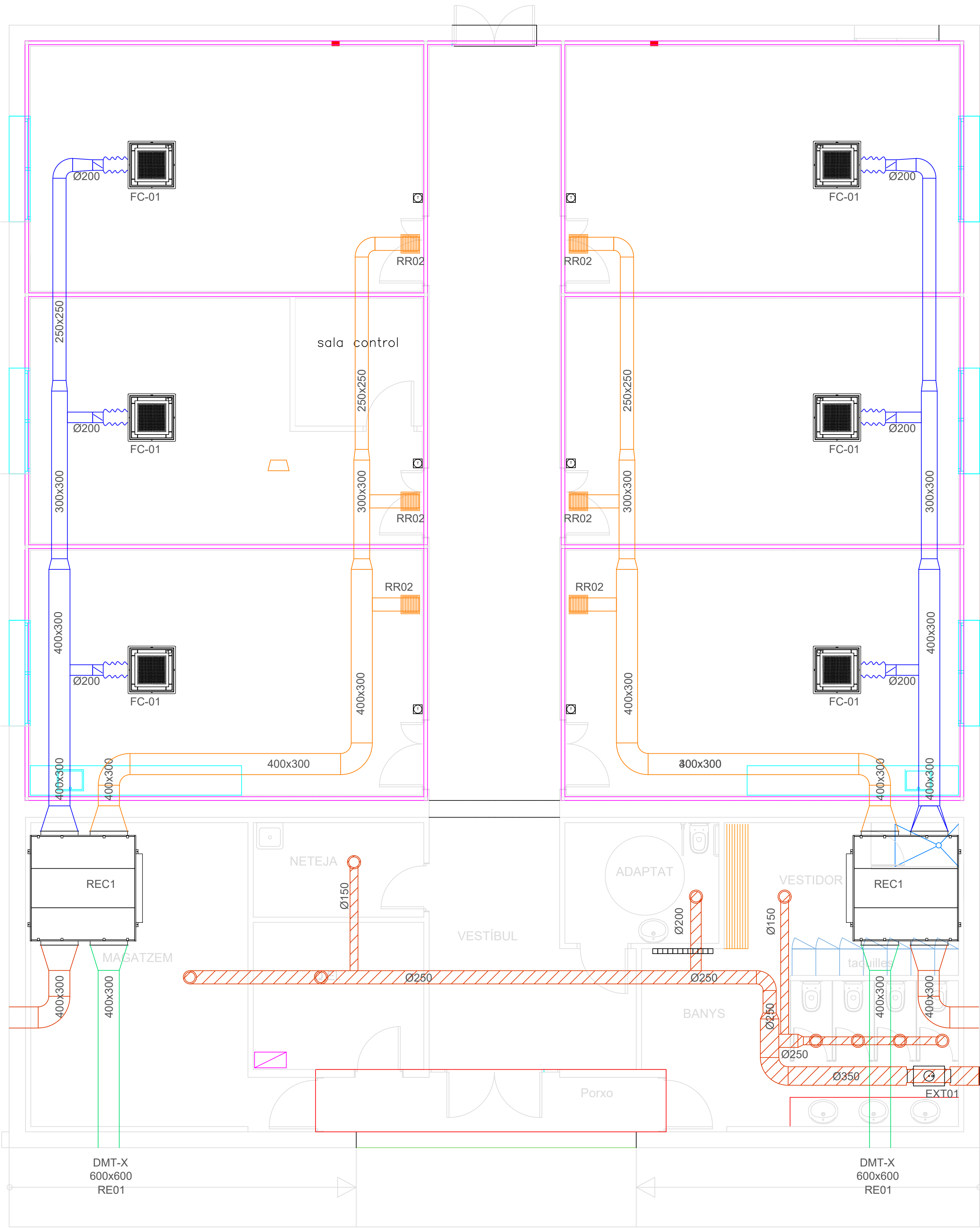
PLANTA BAIXA
