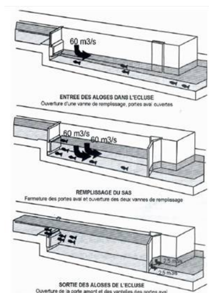
Figura 1. Visió esquemàtica de les fases de funcionament de les resclosos per a navegació adaptades a les necessitats de migració de la saboga (Alosa fallax) al tram inferior del riu Roine (França). Font: Association Migrateurs du Rhône-Méditerranée (2007), a partir de Bechu et al. (1995).
