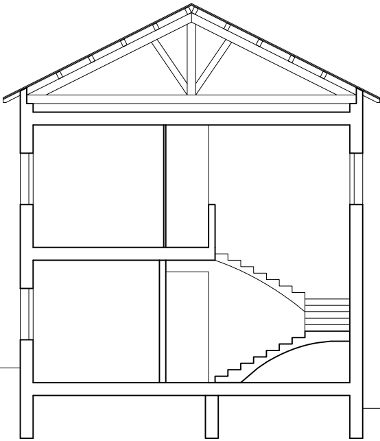
SECCIÓ esc:1/125
