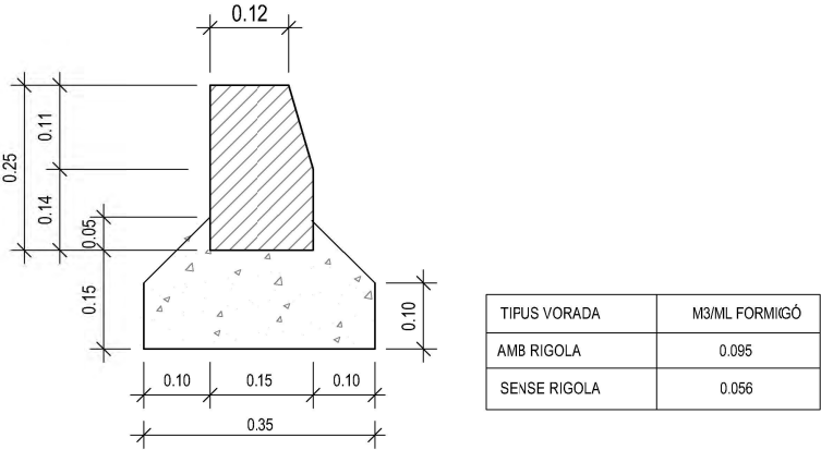
VORADA TIPUS T-2 (NO REMUNTABLE)
