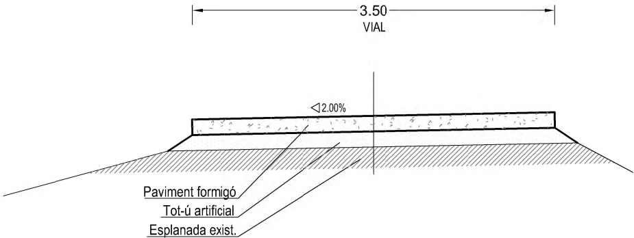
SECCIÓ TIPUS (TRAMS SENSE TALÚS)
