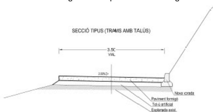
Imatge 3. Detall paviment de formigó
