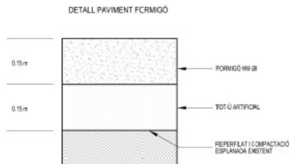
Imatge 4. Detall paviment de formigó
