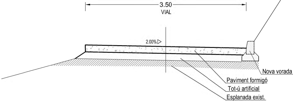
SECCIÓ TIPUS (TRAMS AMB TALÚS)
