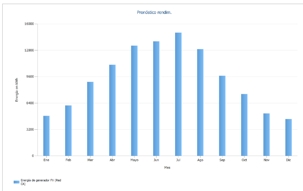
Figura 9. Gràfica de generació elèctrica anual. FONT: PVSOL
