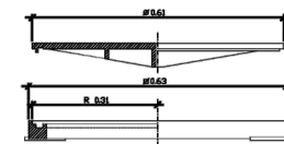
SECCIÓ H-H'
