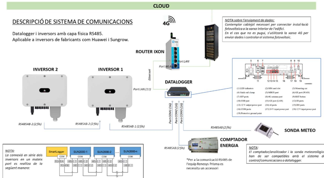
Figura 5 Esquema de comunicacions instal·lacions fotovoltaiques amb RS485. Font: Infraestructures.cat
