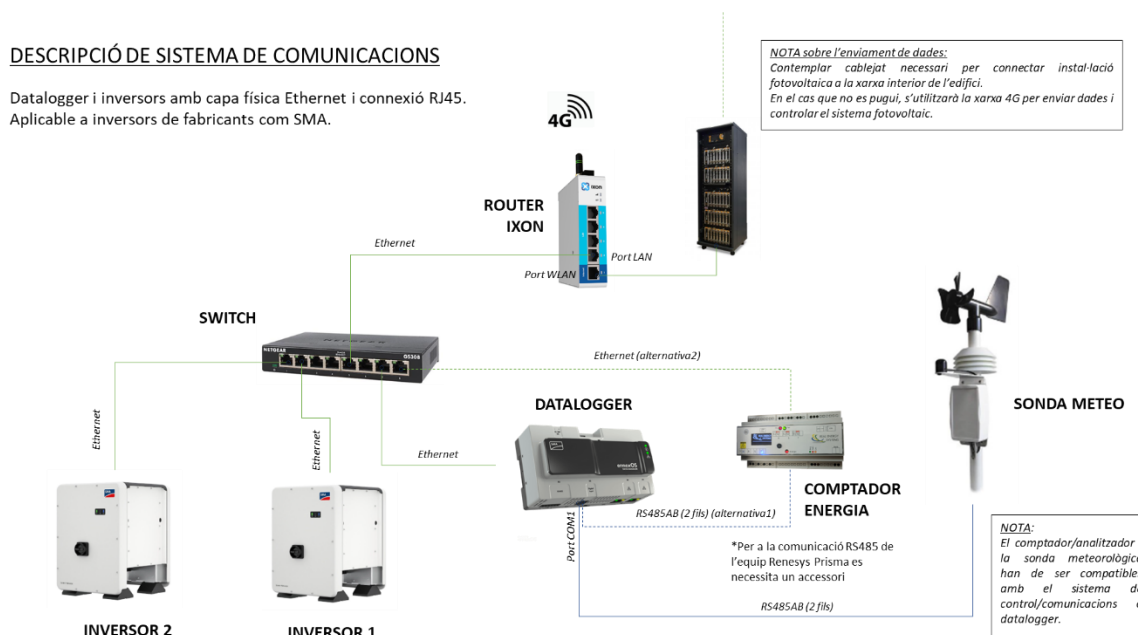
Figura 14 Esquema de comunicacions instal·lacions fotovoltaïques amb Ethernet. Font: Infraestructures.cat
