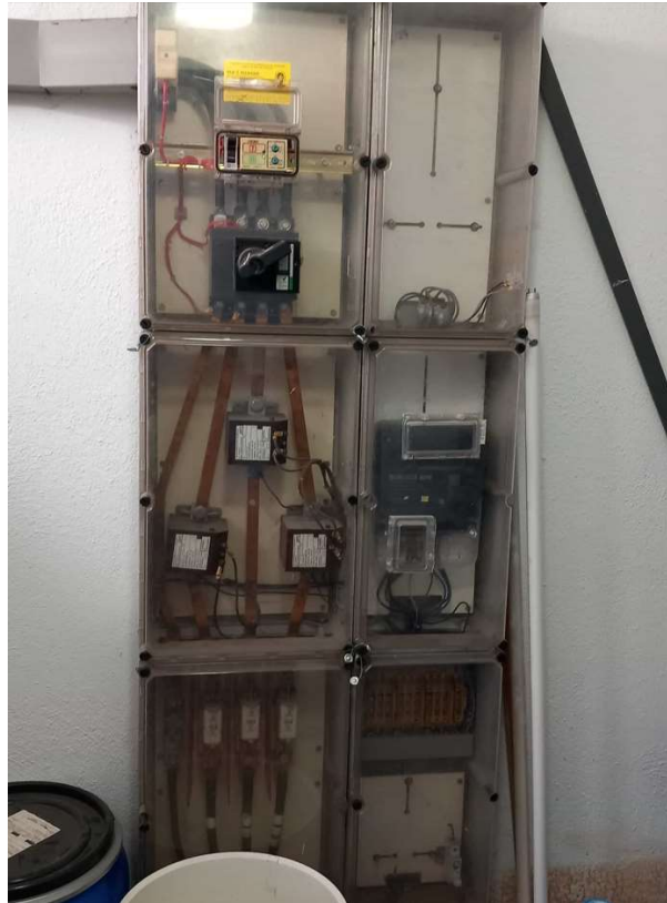
Figura 9 – Ubicació TMF-Consum actual. Font: Infraestructures.cat
