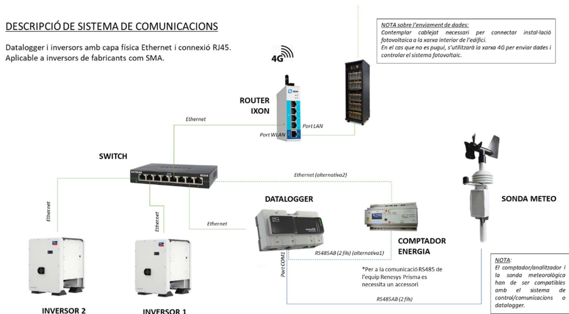
Figura 13 Esquema de comunicacions instal·lacions fotovoltaïques amb Ethernet. Font: Infraestructures.cat
