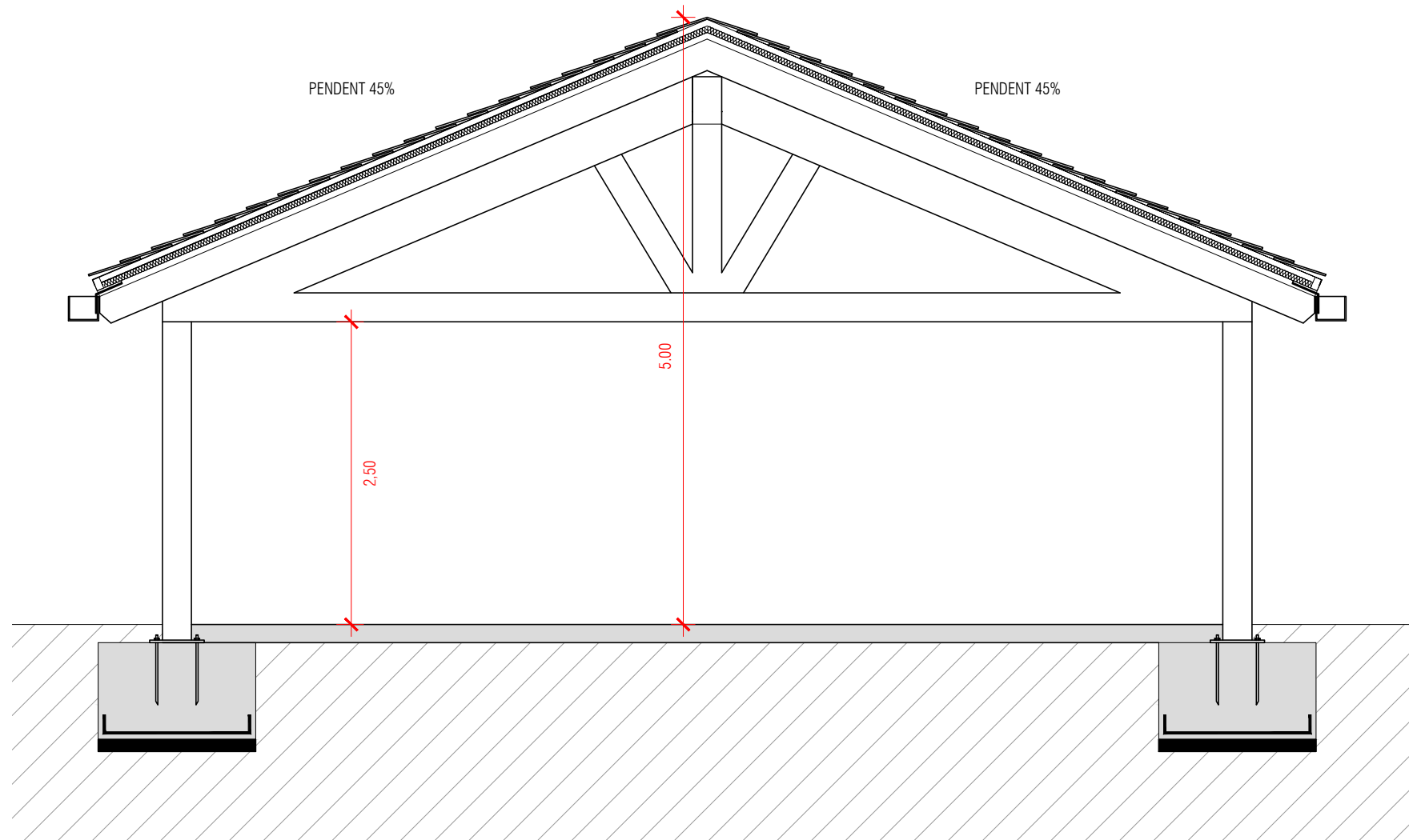
SECCIÓ A-A E./1:50
