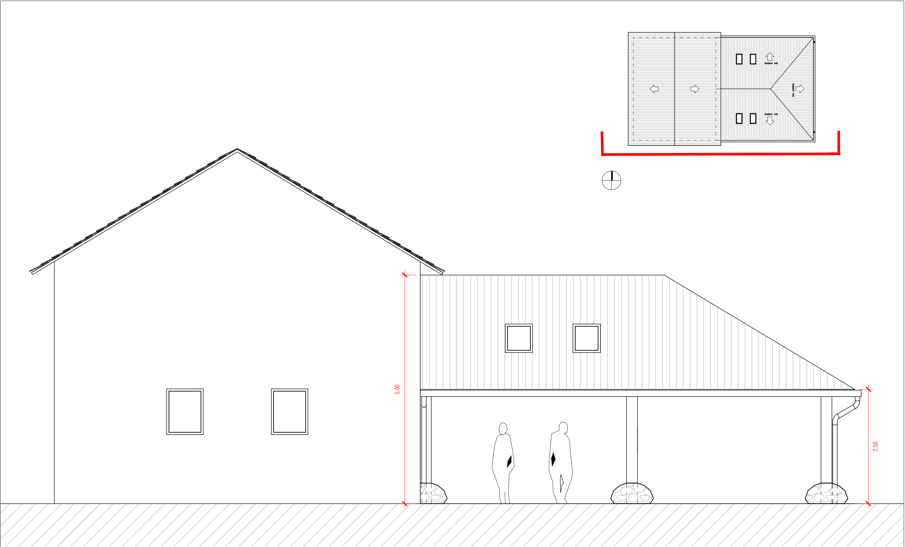
FAÇANA E./1:50
