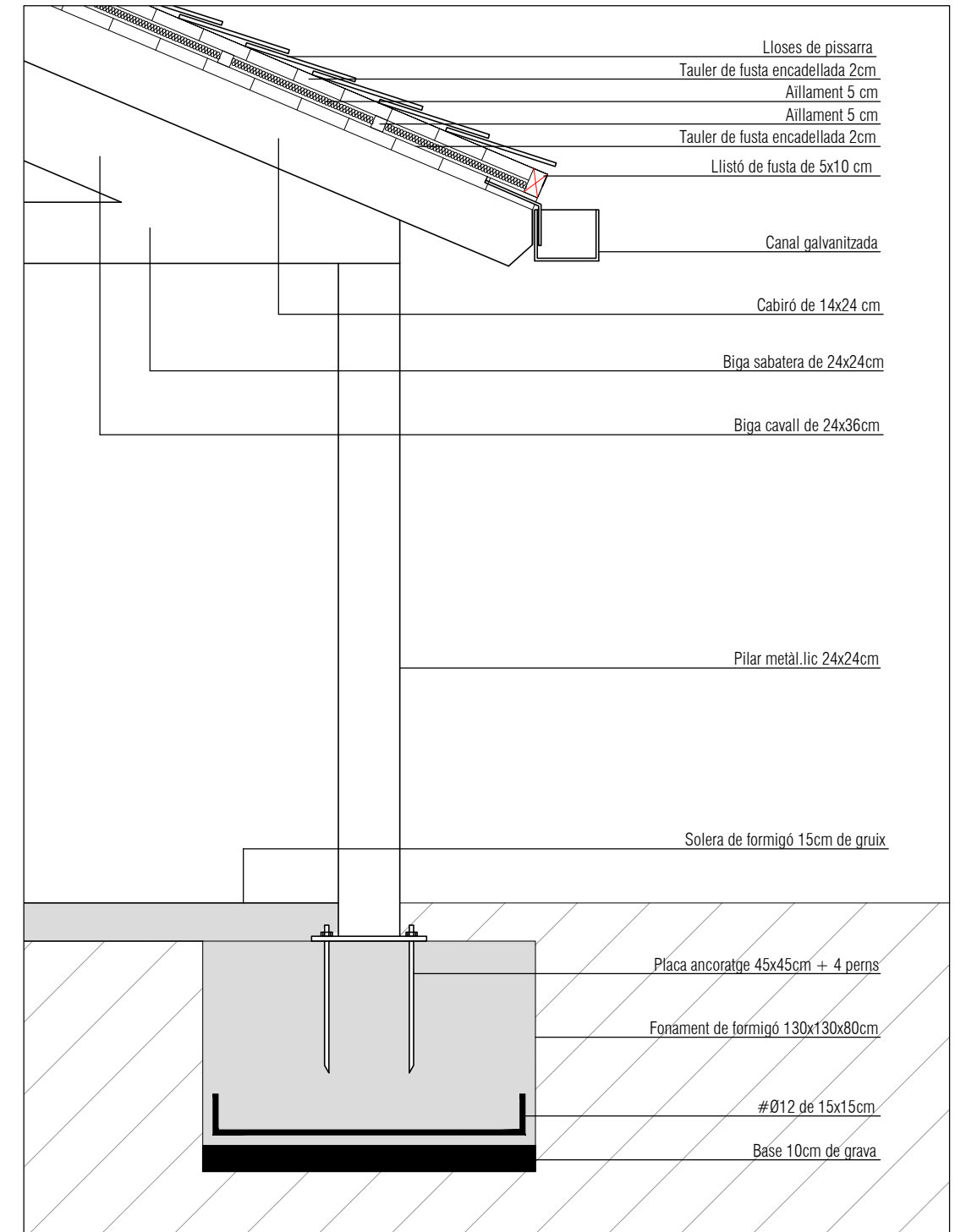
DETALL CONSTRUCTIU E./1:25
