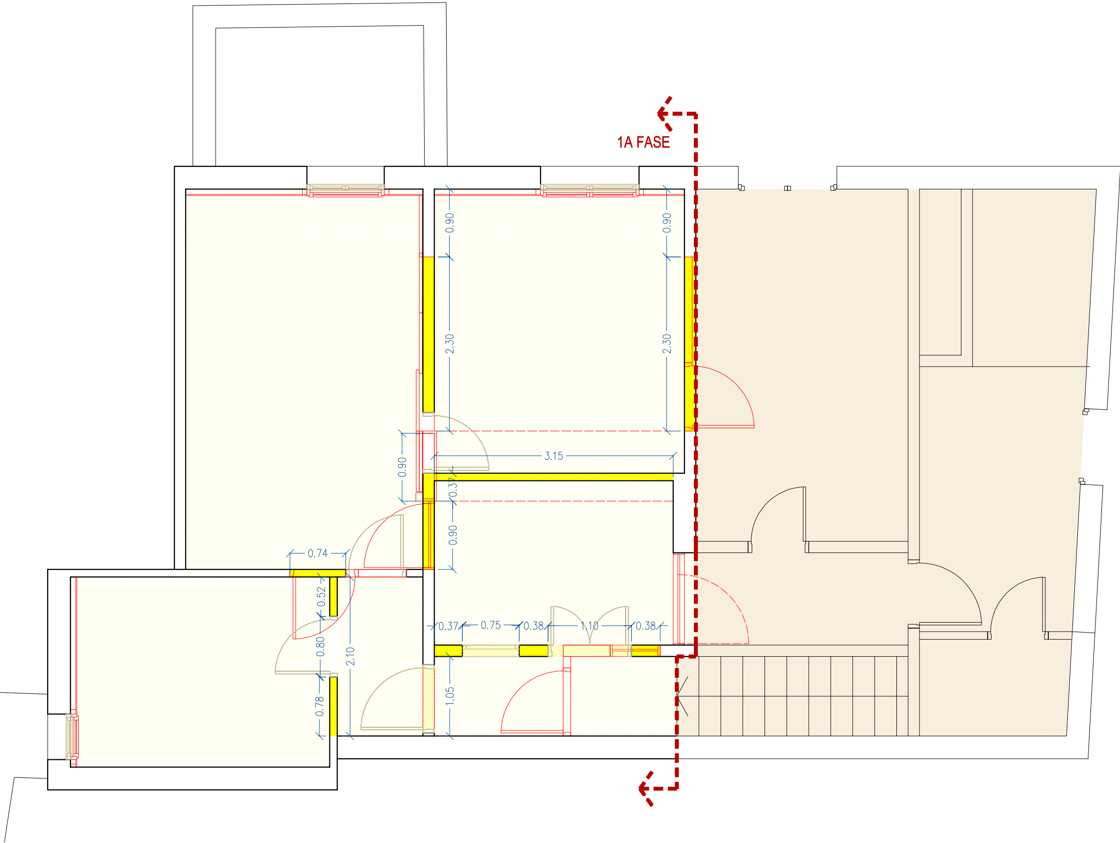
PLANTA DISTRIBUCIÓ OFICINES
