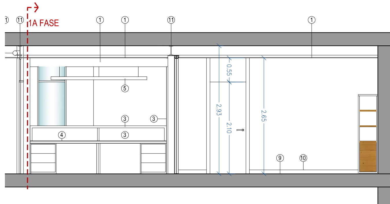
SECCIÓ B
