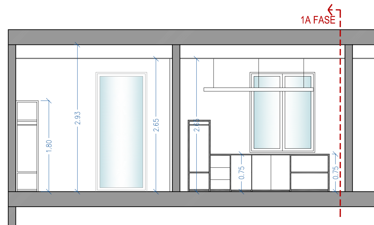
SECCIÓ A
