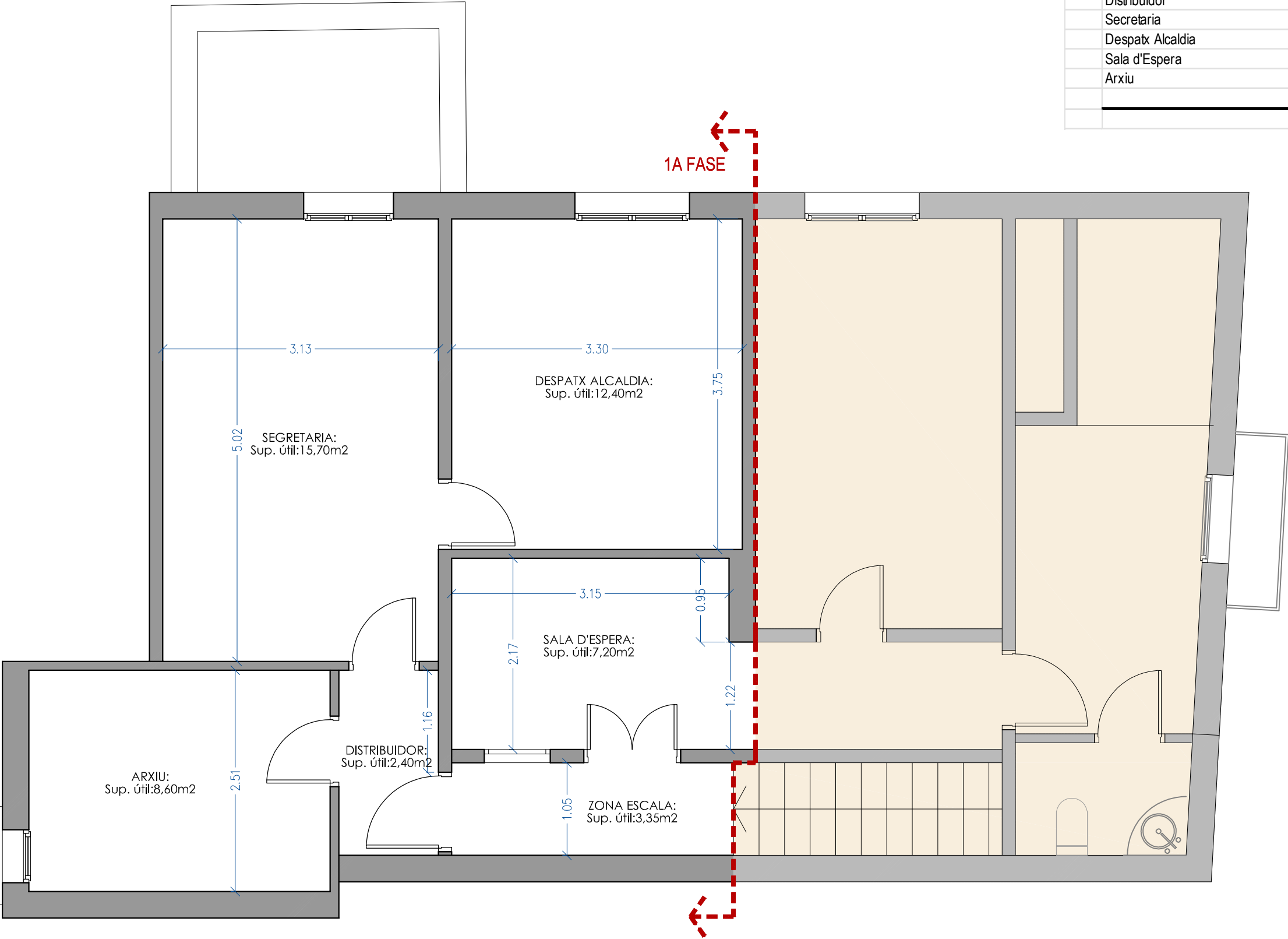
PLANTA DISTRIBUCIÓ OFICINES
