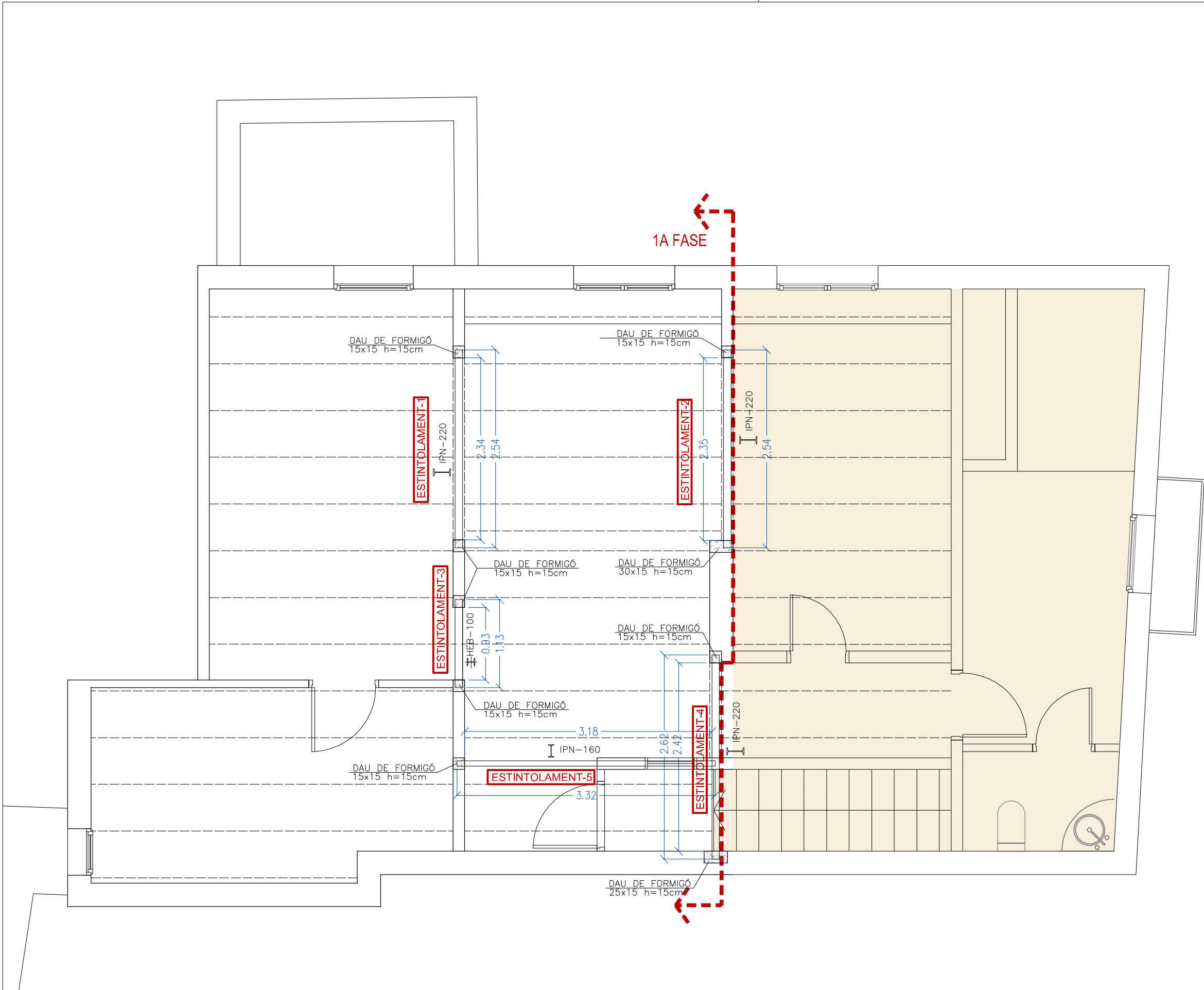
PLANTA DISTRIBUICIÓ OFICINES
