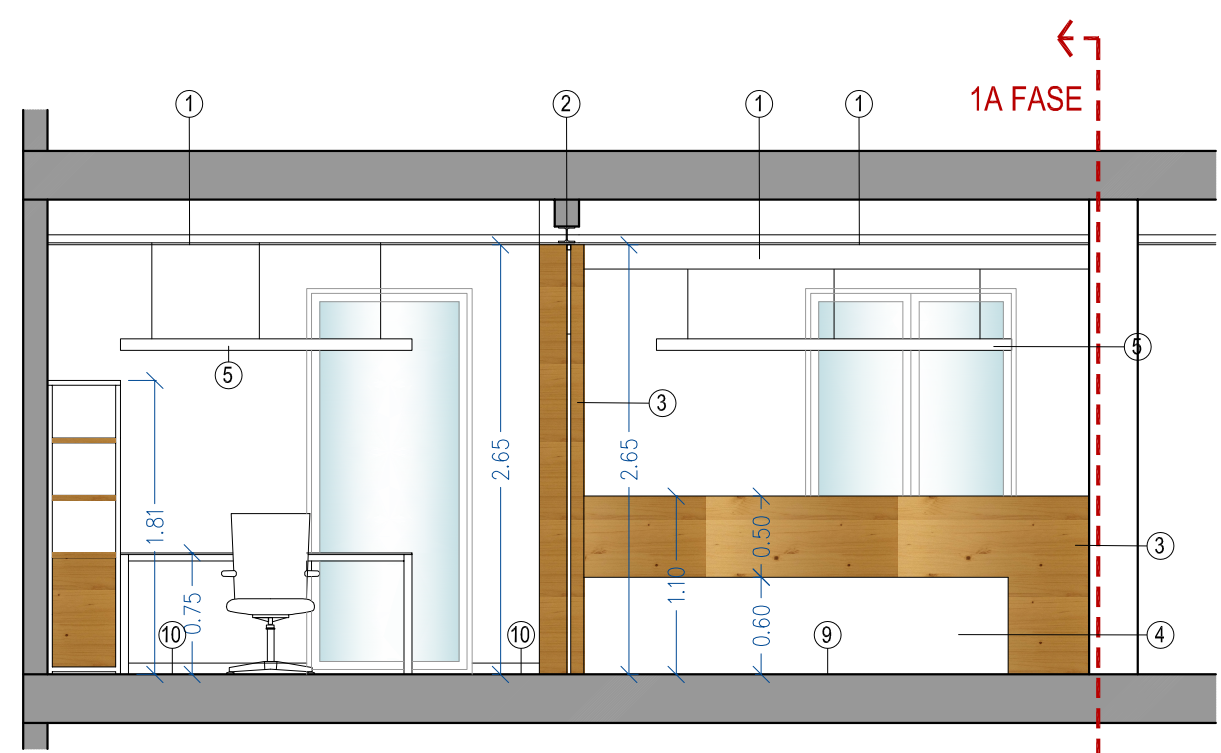
SECCIÓ C
