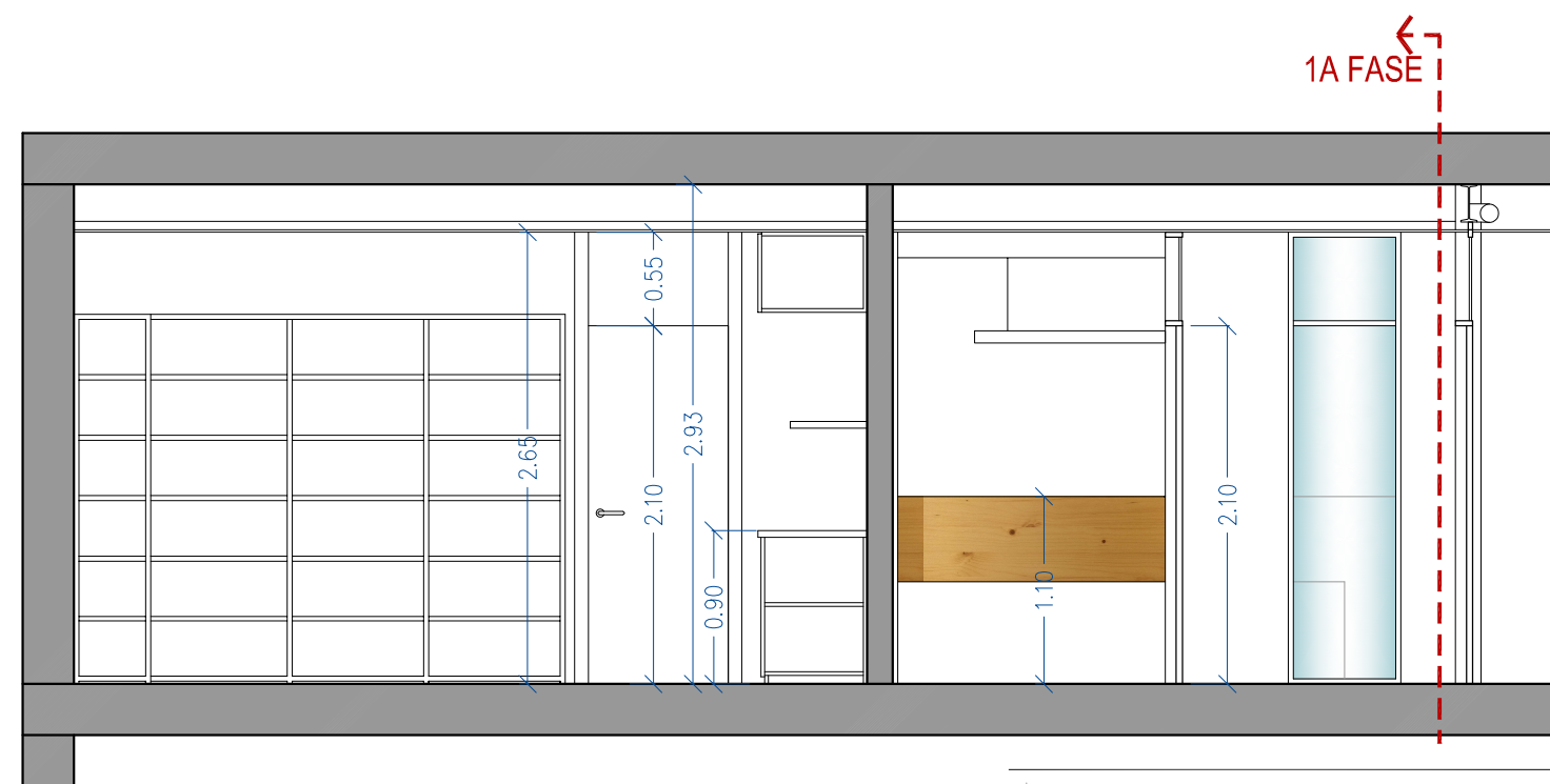
SECCIÓ D
