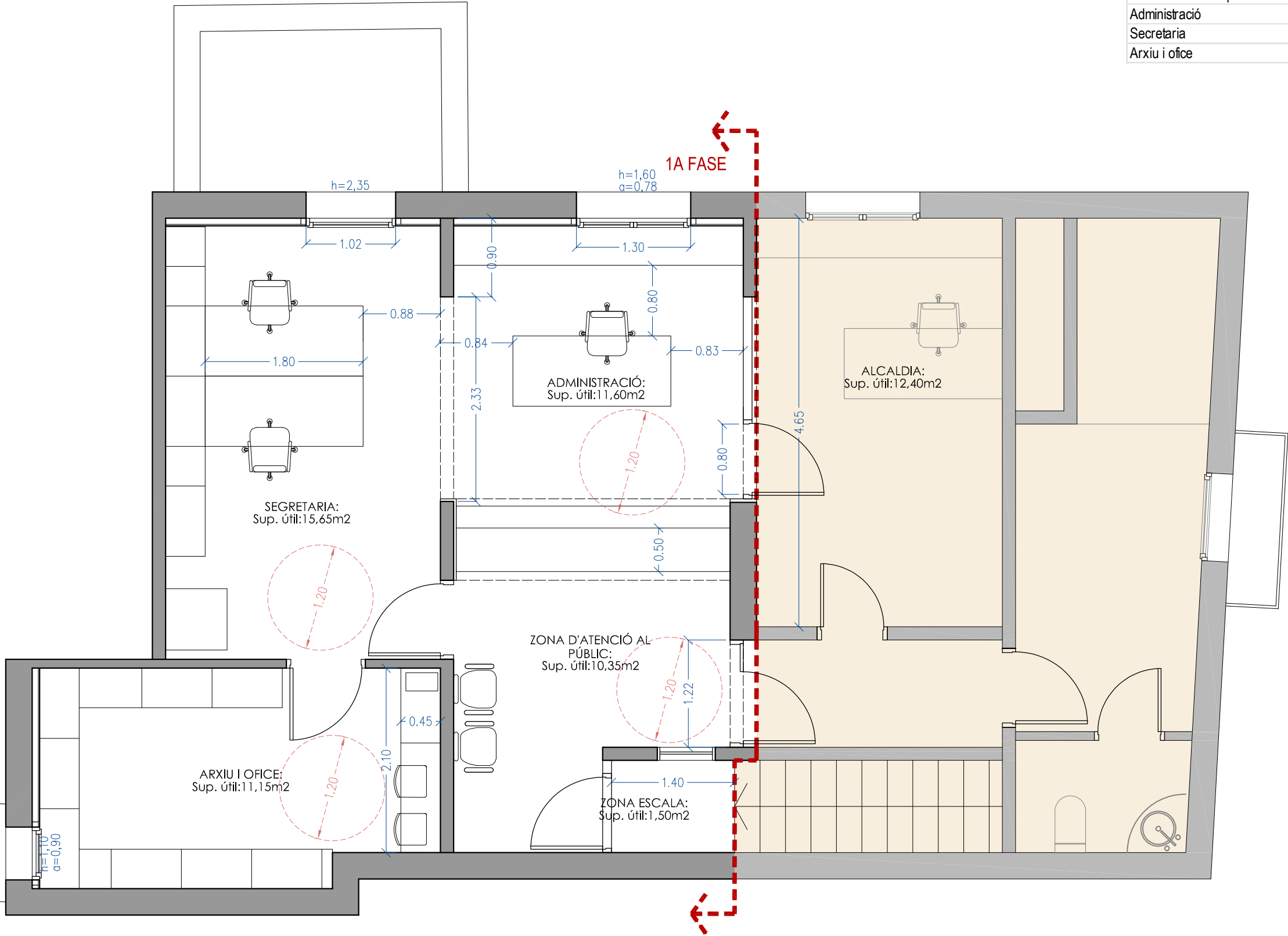
PLANTA DISTRIBUICIÓ OFICINES
