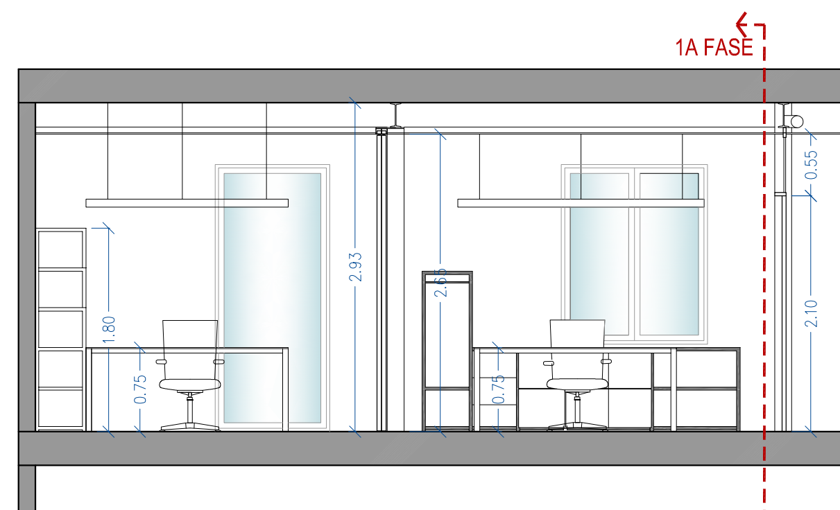
SECCIÓ B
