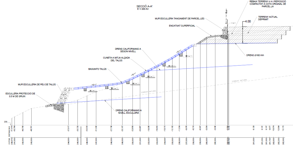
Fig. 2: secció transversal de les obres a realitzar al talús.
