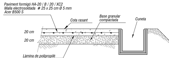
DETALL ACABAT PAVIMENTACIÓ
