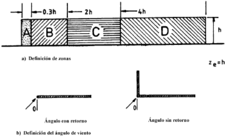
Fig. 10.4.1 – Muros linderos
