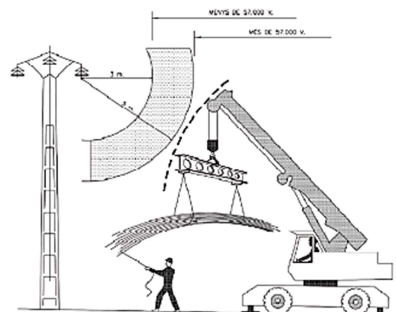
INTERFERÈNCIA DE GRUA AMB LÍNIA ELÈCTRIÇA AÈRIA DE A.T.
