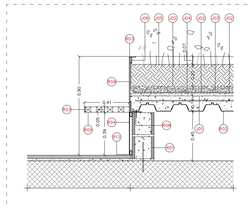
SECCIÓ I-I'
