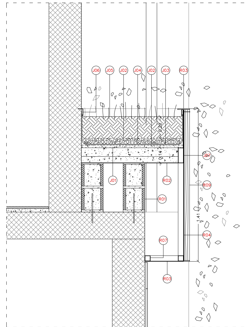
SECCIÓ H-H'
