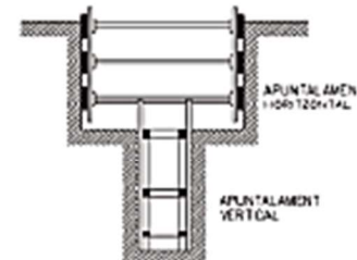
RASA PROFUNDITAT AMB SOBRECÀRREGA
