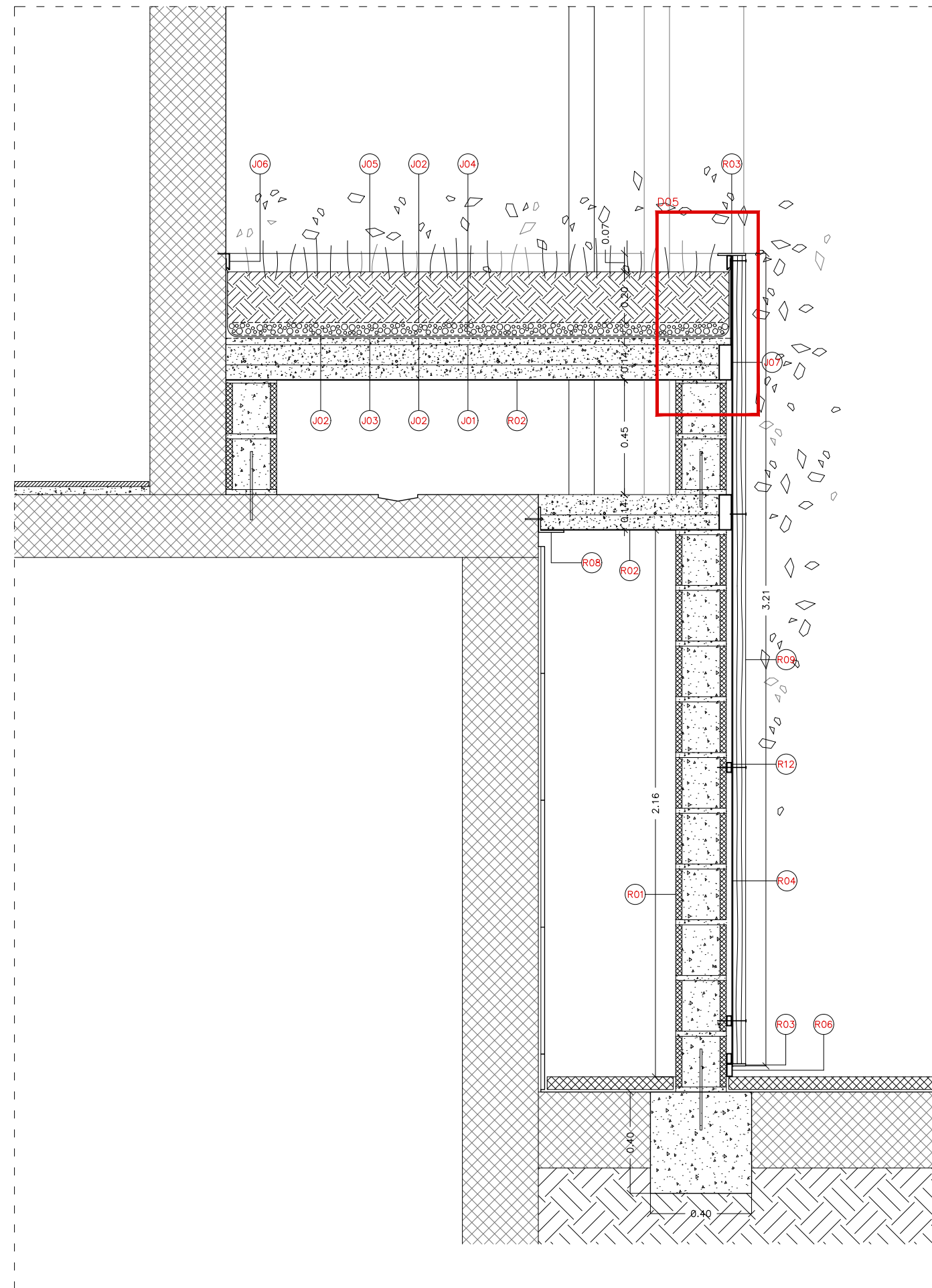
SECCIÓ G-G'
