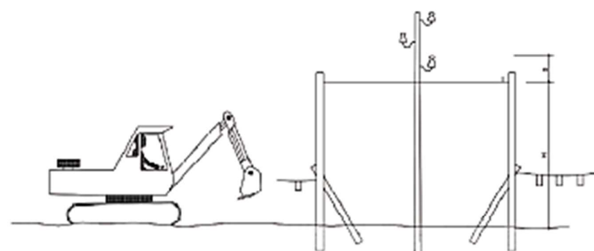
PÒRTIC D'ABALISAMENT DE LÍNIES ELÈCTRIQUES AÈRIES
