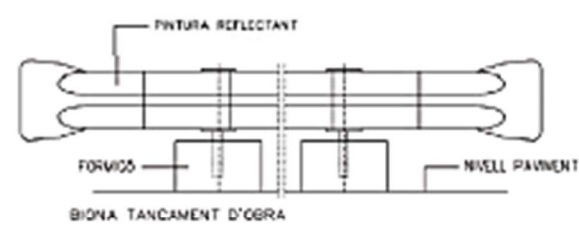
VISTA LATERAL
