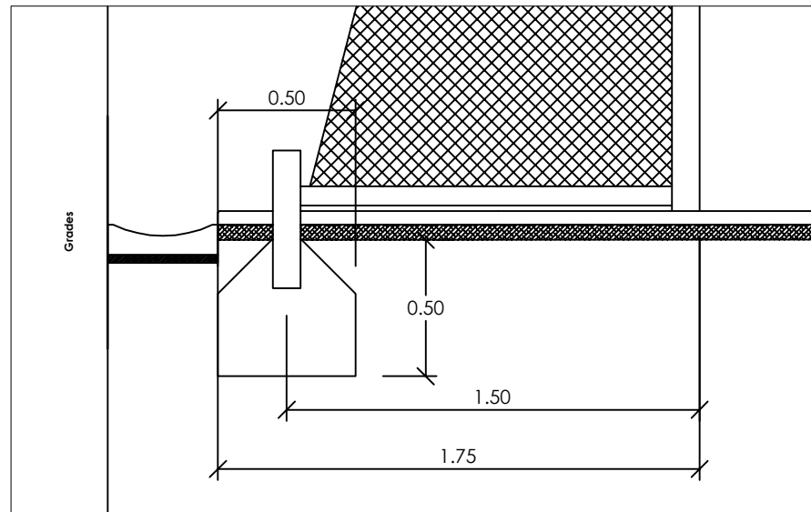
Secció Porteria - Muntanya e: 1/25
