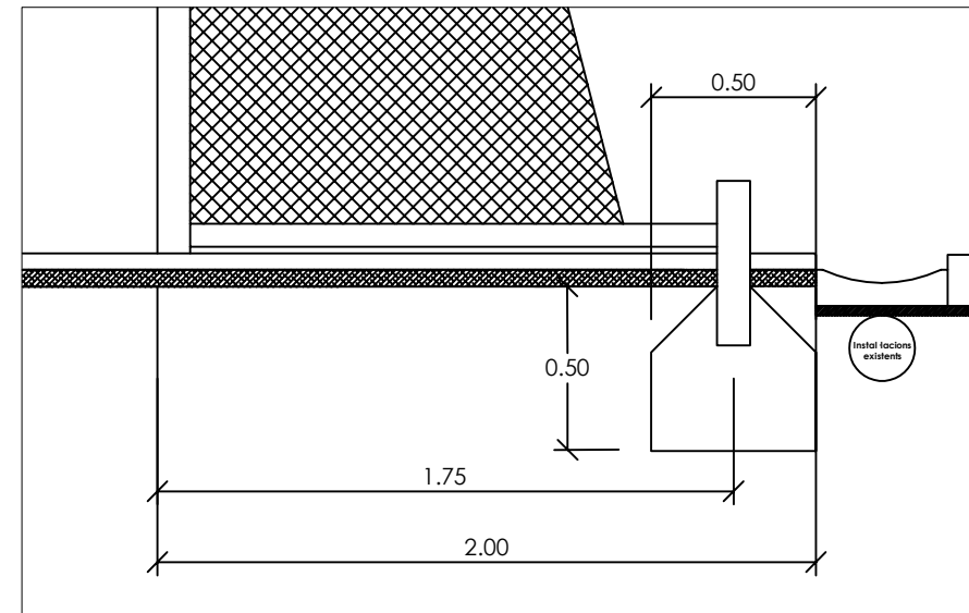
Secció Porteria - Mar e: 1/25
