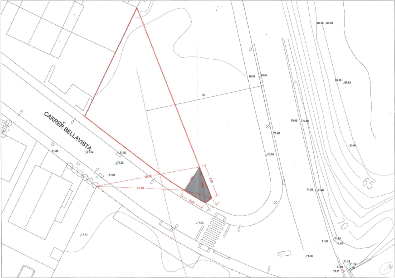
ÀMBIT ESPAI LLIURE Q3.1 E/1:250
